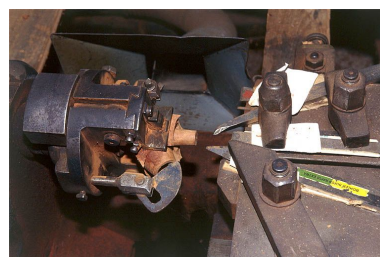
Vue rapprochée du mandrin gueule de loup et des outils. Phot. Jérôme Mongreville IVR43_20003901043ZA
