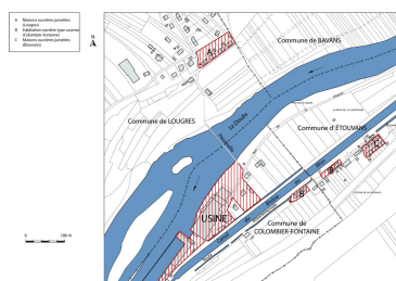
Plan de situation. Montage d'extraits de plans cadastraux numérisés, communes de Colombier-Fontaine et Etouvans (sections A) et Lougres (AE), échelle 1:2500. Dess. Mathias Papigny IVR43_20142500569NUDA
