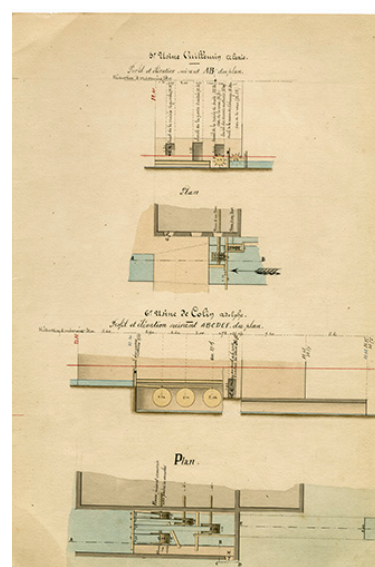
Commune de Grand'Combe. Règlement d'eau des usines [...] Dessins de détails [usines Vuillemin et Colin], 21 juin 1876. Autr. Couturier IVR43_20182500033NUC4A
