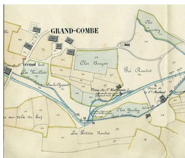
Commune de Grand'Combe. Règlement d'eau des usines [...] Plan parcellaire [détail de la partie centrale : Vermot, Vuillemin et Sudant], 21 juin 1876. Autr. Couturier IVR43_20182500044NUC4A
