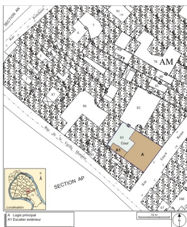
Plan masse et de situation. Extrait du plan cadastral, 1974, section AM. Dess. André Céréza IVR43_20072500010NUDA
