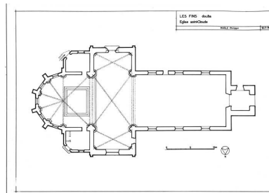
Plan au sol. Phot. Yves Sancey, Autr. Philippe Marle IVR43_19772500282V
