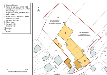
Plan-masse et de situation. Extrait du plan cadastral, 2015, section AC. Dess. Mathias Papigny IVR43_20152502297NUDA
