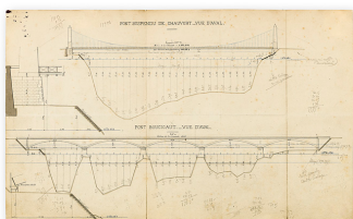
Pont suspendu de Chauvort et pont Me Boucicaut. 1897. Autr. Thevenard, Phot. Thierry Kuntz IVR26_20197100718NUC4A
