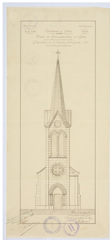
Projet de reconstruction de l'église de Corre. Elévation de la façade principale. [plan, 1897]
