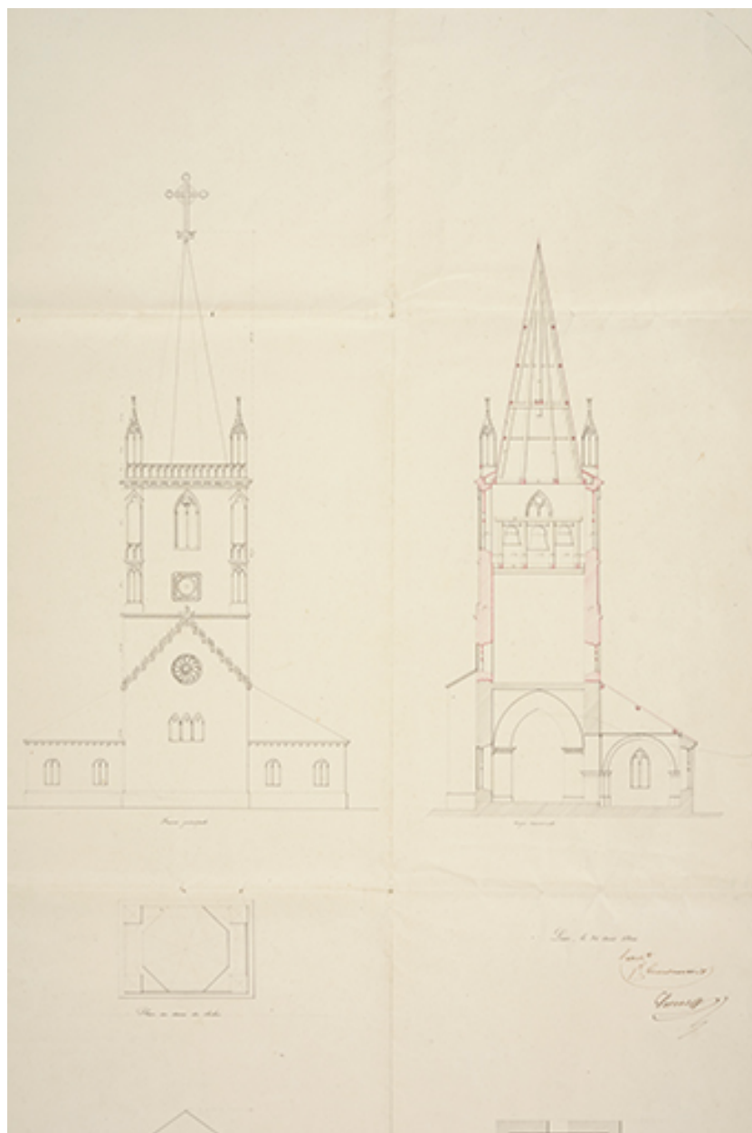
Plan de reconstruction de la partie supérieure du clocher et restauration du chœur de l'église. (détail) 1844
