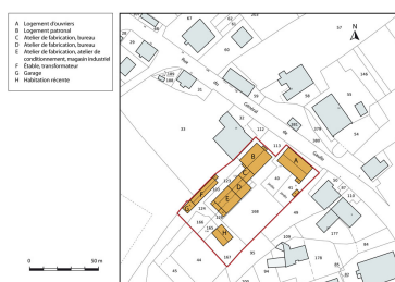
Plan-masse et de situation. Extrait du plan cadastral, 2012, section AB. Dess. Mathias Papigny IVR43_20142501512NUDA
