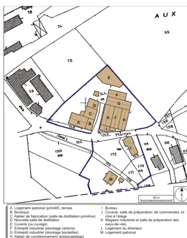
Plan-masse et de situation. Extrait du plan cadastral numérisé, 2008, section AD, 1:1000. Source : Direction générale des Finances Publiques - Cadastre ; mise à jour : 2008. Dess. André Céréza
