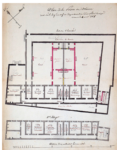
Projet d'extension (plans du rez-de- chaussée et du premier étage). 1835.
