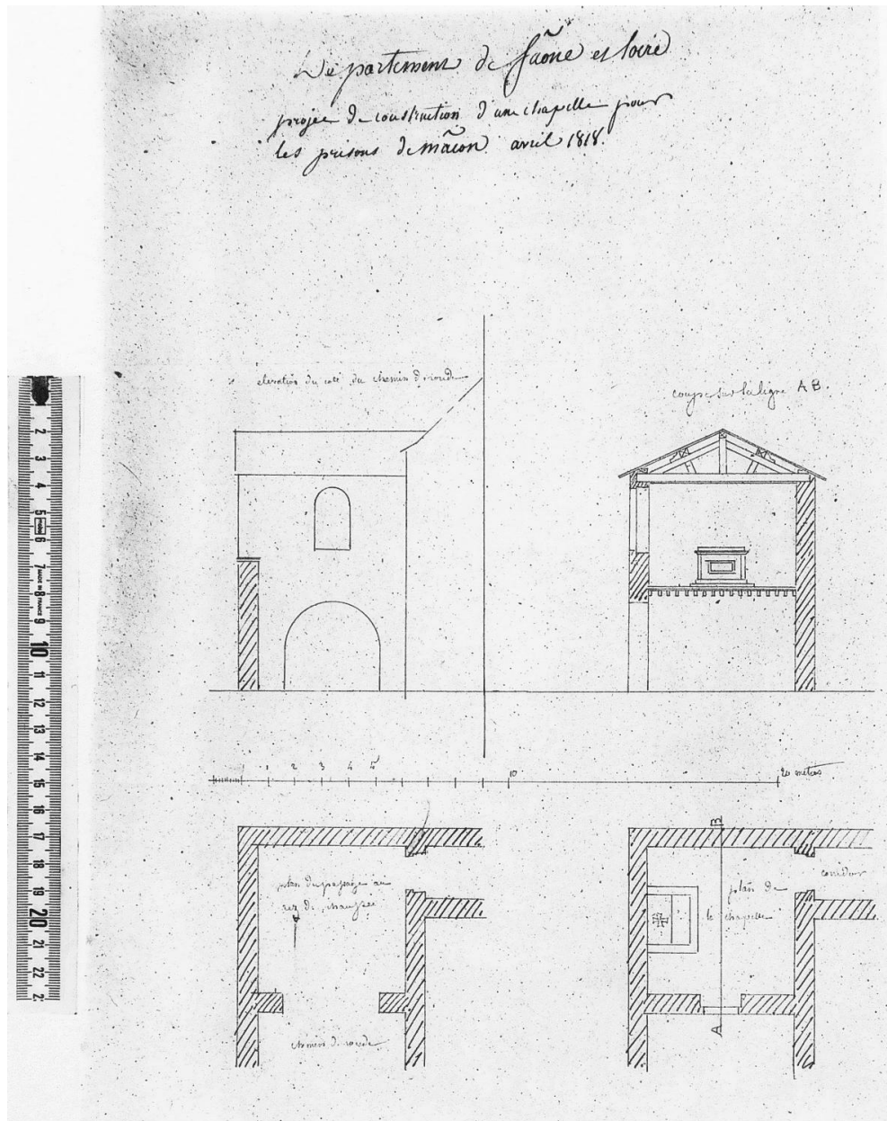
Plans, élévation et coupe de la chapelle. 1818.
