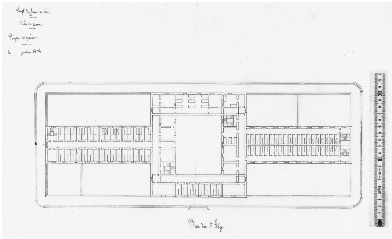
Projet d'extension (plan du premier étage). 1834.
