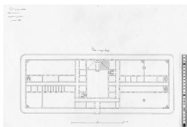
Projet d'extension (plan du rez-de-chaussée). 1834.
