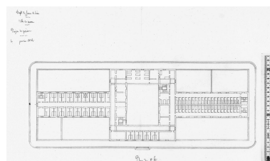
Projet d'extension (plan du premier étage). 1834.
