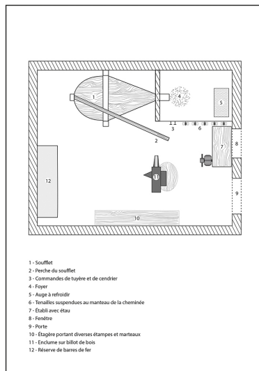
Croquis de plan d'une forge à une fournaise (un poste de travail), [2002]. Dess. Pierre-Marie Barbe-Richaud IVR43_20202500224NUDA
