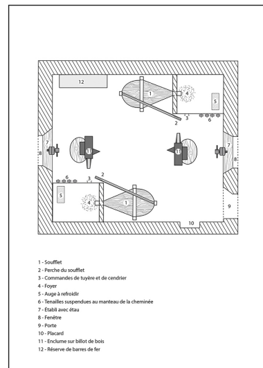
Croquis de plan d'une forge à deux fournaises (deux postes de travail), [2002]. Dess. Pierre-Marie Barbe-Richaud IVR43_20202500225NUDA
