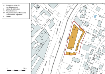
Plan-masse et de situation. Extrait du plan cadastral, 2019. Dess. Bertrand Turina IVR43_20192501086NUDA
