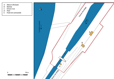
Plan masse et de situation. Dess. Bertrand Turina IVR43_20207000781NUDA
