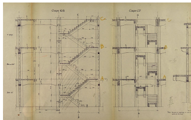
Concours pour la construction d'un entrepôt en béton armé au port de Besançon. Dessins [détail : ] Coupe AB [et] Coupe CD, 1936. Phot. Yves Sancey, Autr. Moreau IVR43_20062500113NUCA
