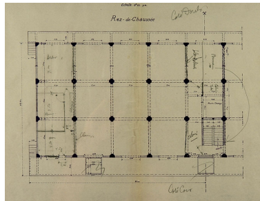
Concours pour la construction d'un entrepôt en béton armé au port de Besançon. Dessins [détail : plan du] Rez-de-chaussée, 1936. Phot. Yves Sancey, Autr. Moreau IVR43_20062500114NUCA
