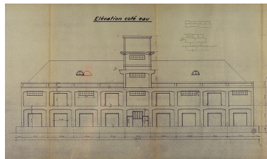
Concours pour la construction d'un entrepôt en béton armé au port de Besançon. Dessins [détail : ] Élévation côté eau, 1936. Phot. Yves Sancey, Autr. Moreau IVR43_20062500111NUCA
