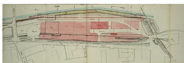
Construction d'un port fluvial à Besançon. Avant- projet. Plan du port, 1933. Phot. Yves Sancey, Autr. Moreau IVR43_20062500057NUCA
