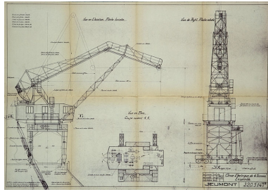
Grue électrique de 4 tonnes. Ensemble, 1936. Phot. Yves Sancey, Autr. Larcier, Autr. Forges et Ateliers de Construction électriques de Jeumont IVR43_20062500058NUCA
