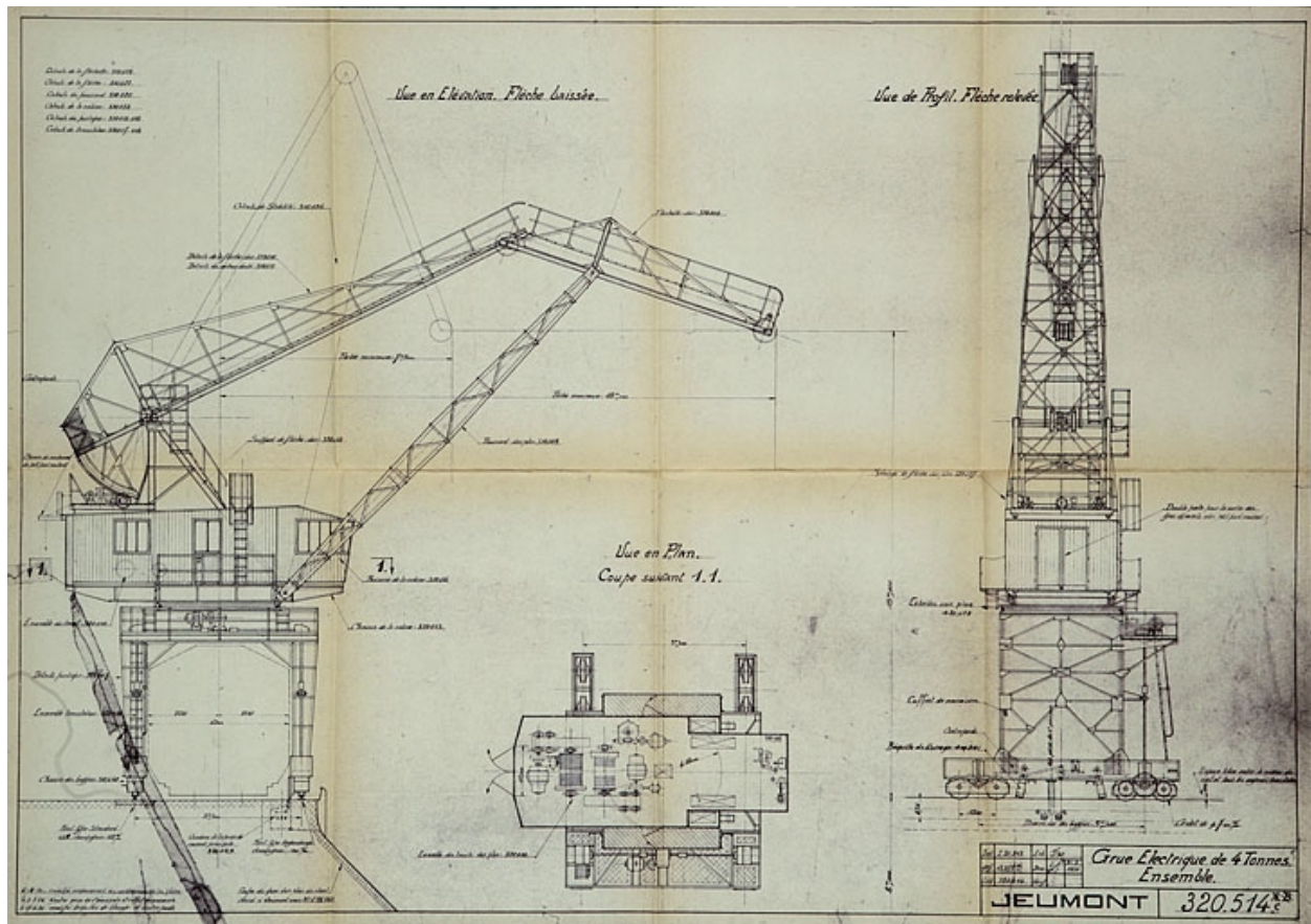
Grue électrique de 4 tonnes. Ensemble, 1936.
