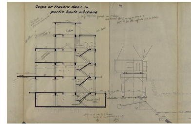
Concours pour la construction d'un entrepôt en béton armé au port de Besançon. Dessins [détail : ] Coupe en travers dans la partie haute médiane, 1936. Phot. Yves Sancey, Autr. Moreau IVR43_20062500115NUCA
