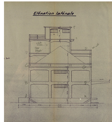
Concours pour la construction d'un entrepôt en béton armé au port de Besançon. Dessins [détail : ] Élévation latérale, 1936. Phot. Yves Sancey, Autr. Moreau IVR43_20062500112NUCA
