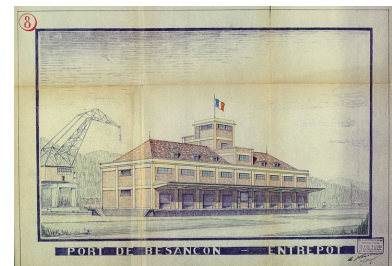
Chambre de Commerce de Besançon. Construction d'un entrepôt en béton armé au port de Besançon. 8. Port de Besançon - Entrepôt [vue perspective], 1936. Phot. Yves Sancey, Autr. S.A. d'Entreprise de Constructions Th. & Ed. Wagner IVR43_20062500076NUCA
