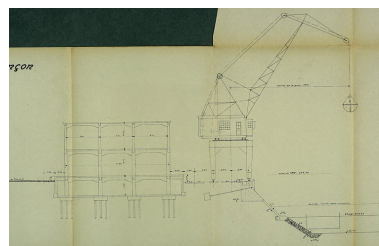
Construction d'un port fluvial à Besançon. Avant-projet. Profil en travers type du port, 1933. Phot. Yves Sancey, Autr. Moreau IVR43_20062500077NUCA
