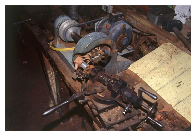
Machine à fraiser. Phot. Jérôme Mongreville IVR43_20003901061ZA
