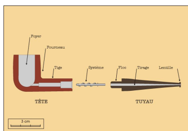
Coupe d'une pipe avec désignation de ses différentes parties.
