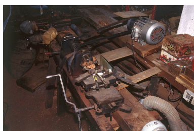
Machine à tourner dite machine à ébaucher. Phot. Jérôme Mongreville IVR43_20003901069ZA
