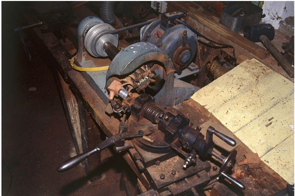
Machine à fraiser.
