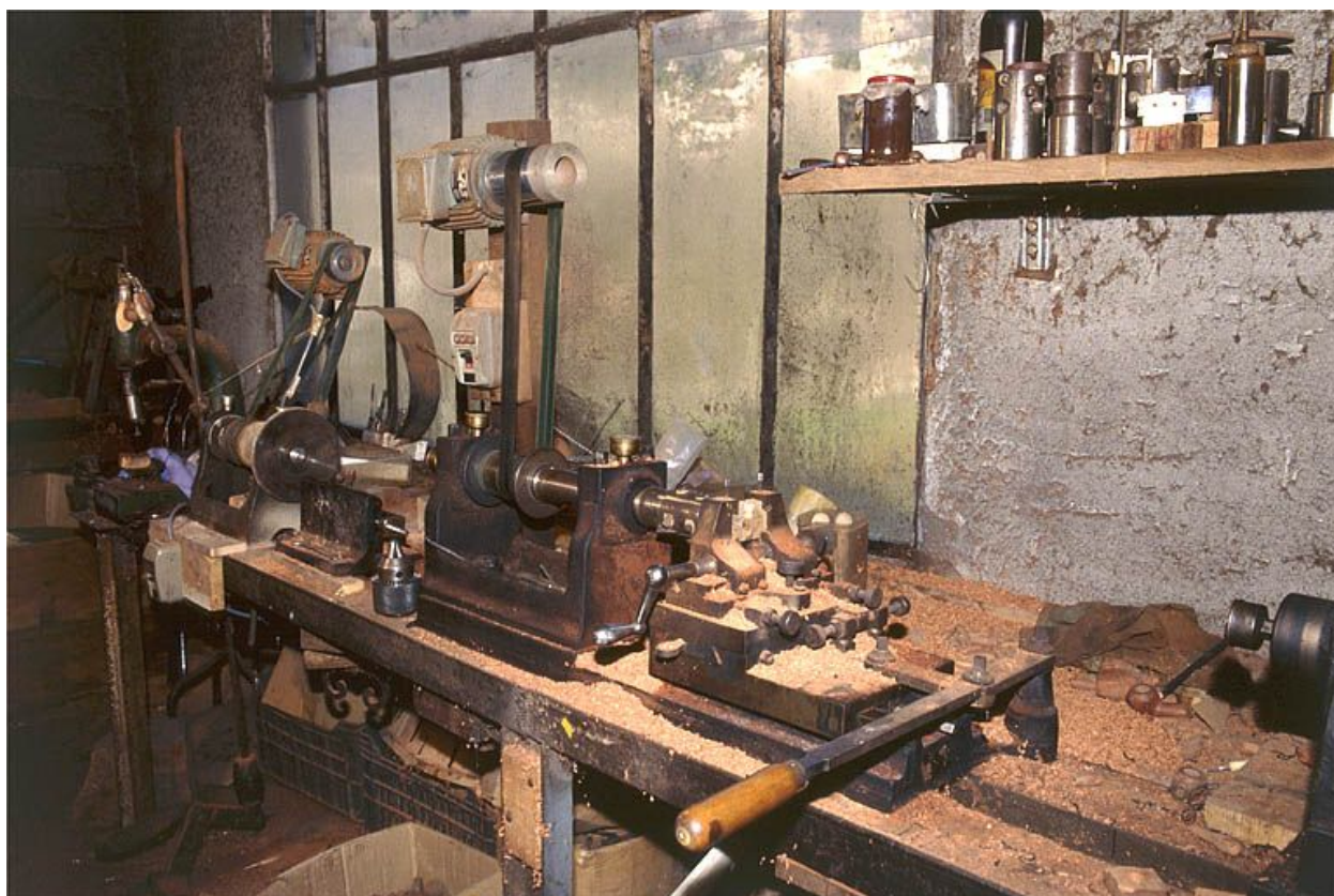
Machine à percer et à fraiser.
