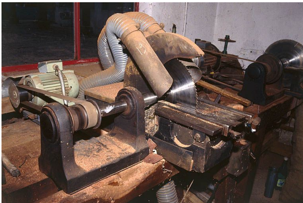
Vue d'ensemble de la scie de gauche, servant au calibrage (dressage des côtés).
