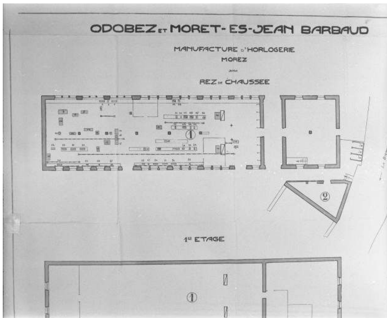
Odobet et Moret-és-Jean-Barbaud. Manufacture d'horlogerie. Morez. [Détail du] Rez de chaussée. Dessin, 1927. Echelle 1:100.
