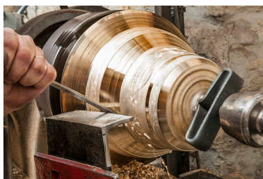
Fonderie de cloches Charles Obertino à Labergement-Sainte- Marie : tournage d'une cloche. Phot. Jérôme Mongreville IVR43_20152502451NUC4A
