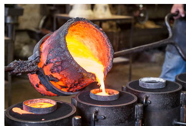
Fonderie de cloches Charles Obertino à Labergement-Sainte-Marie : coulée d'une poche de bronze. Phot. Jérôme Mongreville IVR43_20152502467NUC4A
