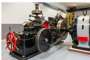
Centrale hydroélectrique du Fourpéret, à Labergement-Sainte-Marie : régulateur de la Société alsacienne de constructions mécaniques.
