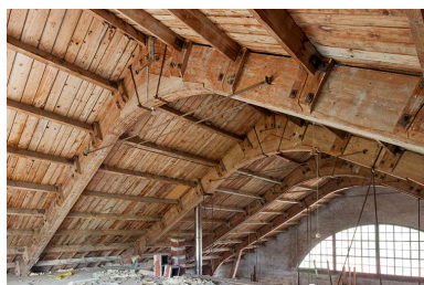
Scierie communale de Remoray- Boujeons. Charpente en bois lamellée-boulonnée. Phot. Jérôme Mongreville IVR43_20152501895NUC4A
