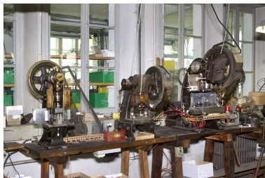
2e, 3e et 4e presses. De gauche à droite : presse Bréguet Frères, presse sans nom et presse Richert-Laval type Perla. Phot. Yves Sancey IVR43_20103900261NUC2A
