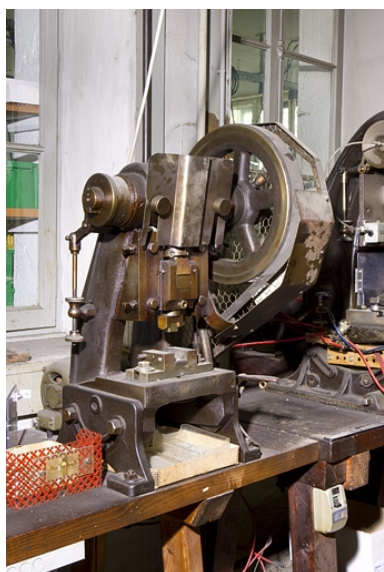
3e presse (sans nom). Phot. Yves Sancey IVR43_20103900263NUC2A
