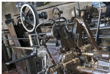
Atelier primitif. Partie supérieure d'une machine à décolleter. Phot. Jérôme Mongreville IVR43_20112501470NUC4A
