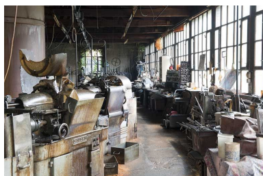
Atelier de décolletage primitif. Vue d'ensemble depuis le sud. Phot. Jérôme Mongreville IVR43_20112501476NUC4A
