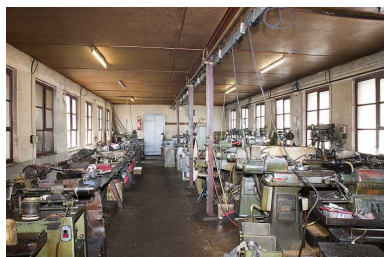
Atelier de décolletage sud. Vue d'ensemble. Phot. Jérôme Mongreville IVR43_20112501479NUC4A
