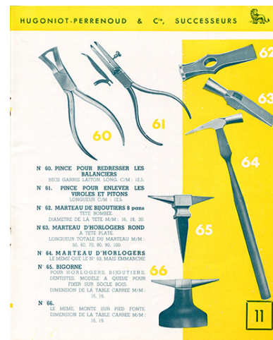
Catalogue L.H.T. 3 [catalogue de production p. 11 : pinces, marteaux et bigornes], [1949].
