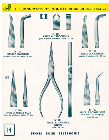
Catalogue L.H.T. 3 [catalogue de production p. 14 : pinces pour téléphonie], [1949]. IVR43_20192500983NUC4A
