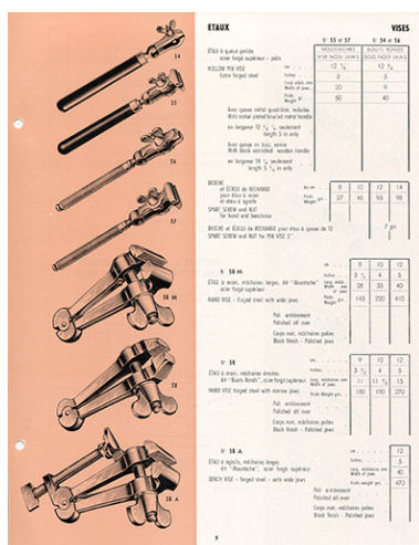
Catalogue L.H.T. 4. [catalogue de production p. 9 : étaux], [3e quart 20e siècle]. IVR43_20192500987NUC4A
