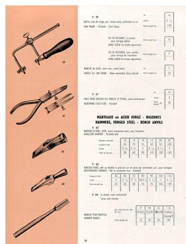
Catalogue L.H.T. 4. [catalogue de production p. 10 : bocfil, pinces et marteaux], [3e quart 20e siècle]. IVR43_20192500988NUC4A
