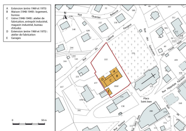
Plan-masse et de situation, avec datation. Dess. Mathias Papigny IVR43_20162501507NUDA
