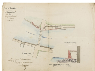
Pont de Pontailleur. Plan général. Projet d'une banquette de halage.
