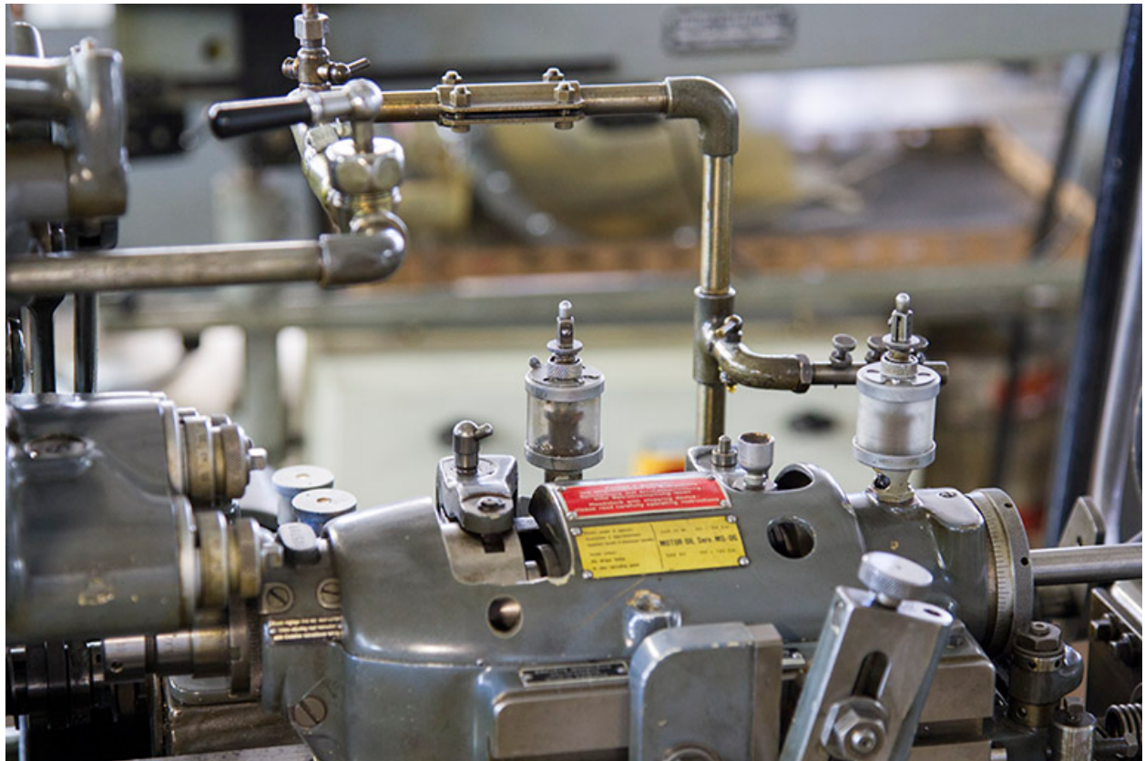
Le système de lubrification.
