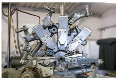
La lunette à bascule, avec ses cinq porte-burins. Phot. Jérôme Mongreville IVR43_20142500723NUC2A
