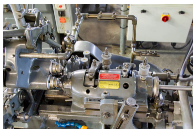
Vue plongeante sur la poupée mobile et le système de lubrification. Phot. Jérôme Mongreville IVR43_20142500718NUC2A
