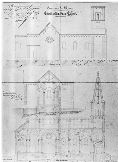
Elévation latérale, coupe transversale et coupe longitudinale. Phot. Yves Sancey, Phot. Achille Paillot IVR43_19833900775V
