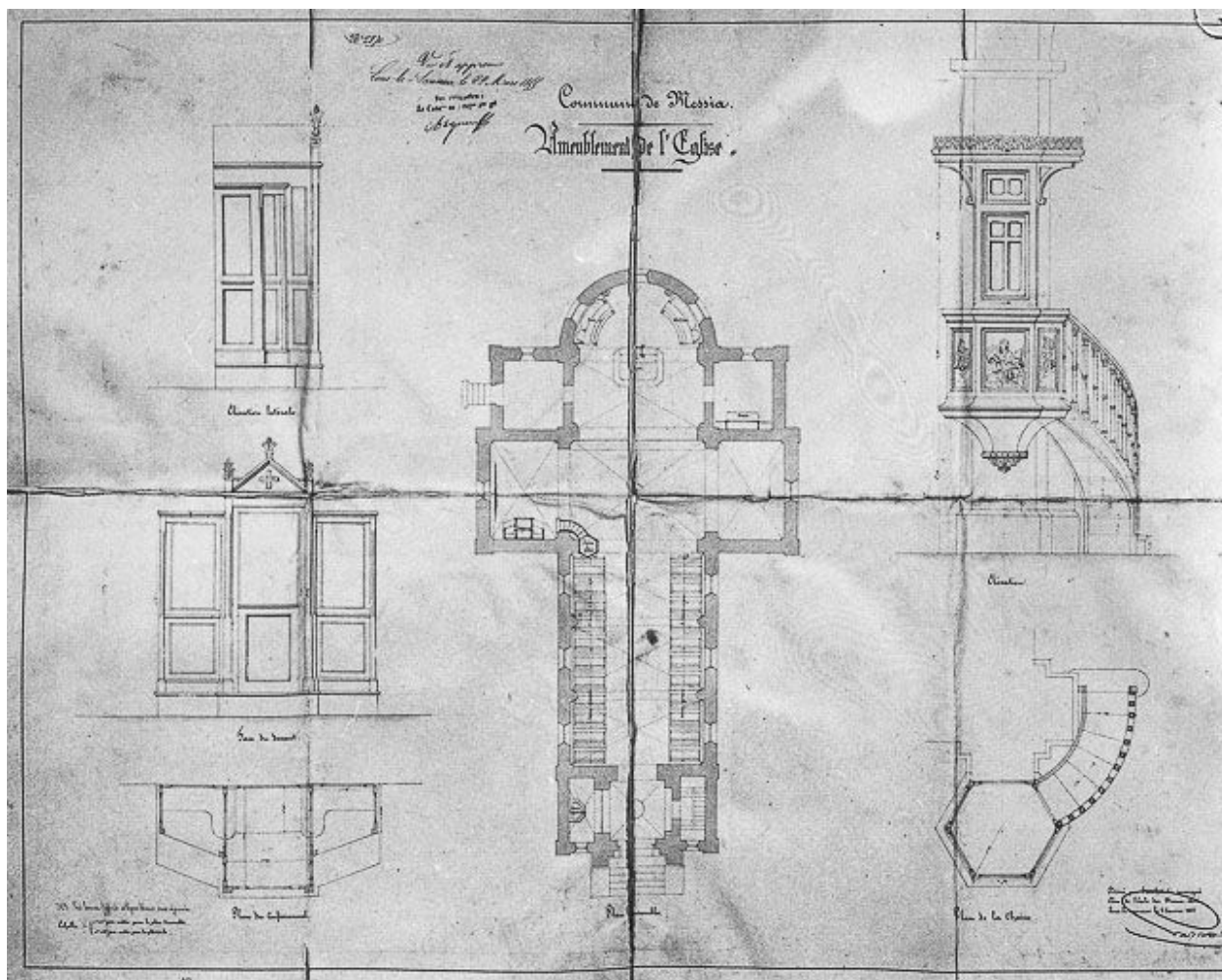
Ameublement de l'église : plan général, confessionnal, chaire.
