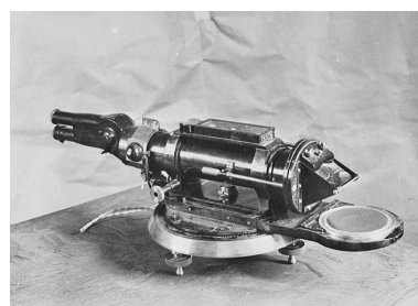
[Astrolabe à prisme avec micromètre enregistreur], 1ère moitié 20e siècle. Cet instrument est-il celui mis au point par Claude et Driencourt en 1905 ? Phot. Yves Sancey IVR43_20042500159X
