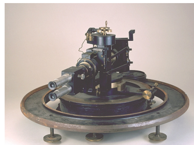
Vue d'ensemble, côté objectif. Phot. Jérôme Mongreville IVR43_20032501007XA
