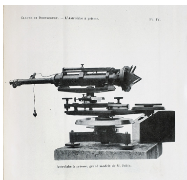
Astrolabe à prisme, grand modèle de M. Jobin, 1910. Phot. Yves Sancey IVR43_20072500861NUCA
