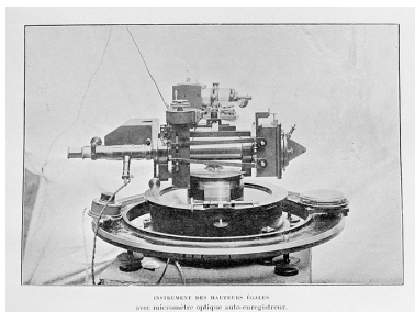
Instrument des hauteurs égales avec micromètre optique auto-enregistreur, 1936. Phot. Yves Sancey IVR43_20042500194X
