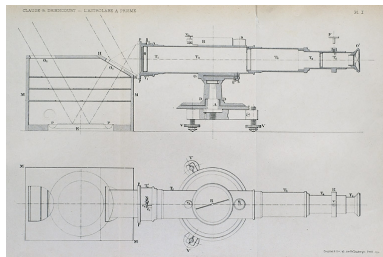
[Astrolabe à prisme Claude et Driencourt : coupe verticale et coupe horizontale], 1910. Phot. Yves Sancey, Autr. Courtier et Cie IVR43_20072500858NUCA
