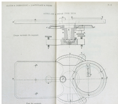
[Astrolabe à prisme Claude et Driencourt : coupe verticale et plan du support], 1910. Phot. Yves Sancey, Autr. Courtier et Cie IVR43_20072500859NUCA
