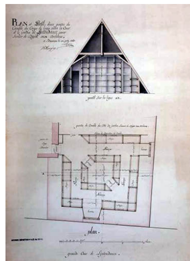
Plan et profil d'une partie du comble du corps de logis entre cour et jardin. Dessin à la plume aquarellé, 30 juin 1758.
