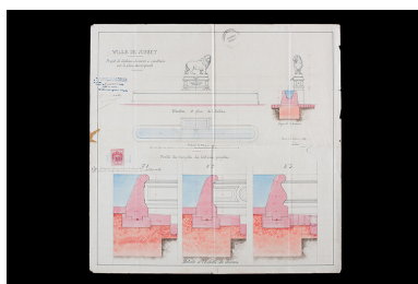
Élévation, profil, plan et coupe de la fontaine, 1869. Phot. Nicolas Waltefaugle IVR43_20257000193NUC4A
