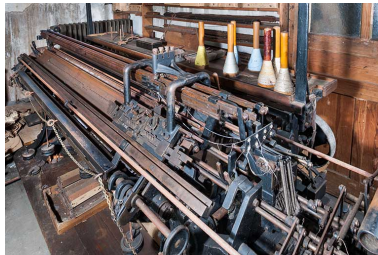
Machine à tricoter à plat (détail). Phot. Jérôme Mongreville IVR43_20142500225NUC4A
