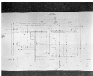
Section de Taillat (les Bouchoux). Construction d'une porcherie. Plan de l'établissement. Phot. Jérôme Mongreville IVR43_19943901390X
