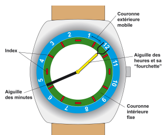
Schéma du cadran et des organes d'affichage.
