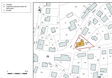
Plan-masse et de situation. Extrait du plan cadastral, 2015, section AD. Dess. Mathias Papigny IVR43_20152500658NUDA
