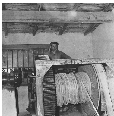
Tirage d'un bloc sur le chantier : le treuil. Phot. Yves Sancey IVR43_19973900018X
