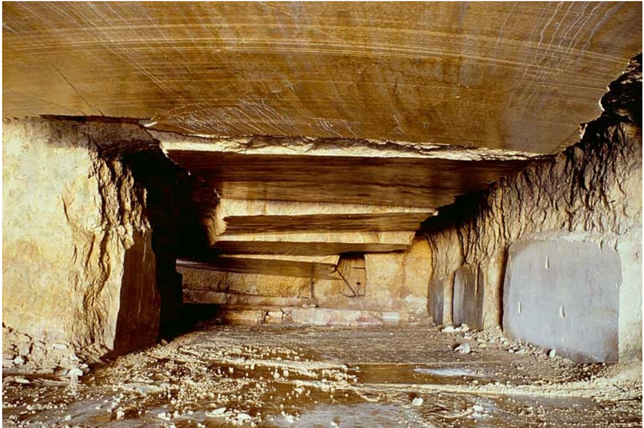
Intérieur, partie centrale, depuis une entrée. Au fond à droite, poulies de renvoi du fil hélicoïdal.
