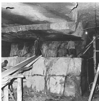
Intérieur de la carrière : fil hélicoïdal en place après dégagement des stériles.
