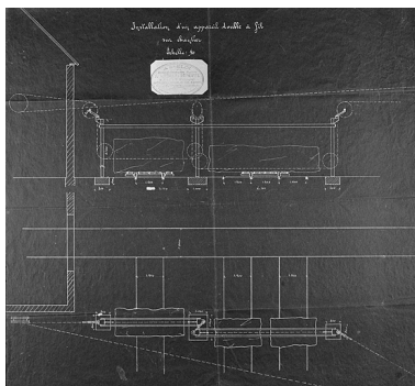
Installation d'un appareil double à fil sur chantier [projet]. Phot. Yves Sancey, Autr. Thonar Dejaiffe IVR43_19973900020X
