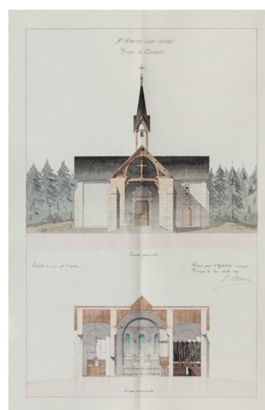
Projet d'Émile Tarlier (1871), élévation et coupe transversale. Repro. Pierre-Marie Barbe- Richaud, Autr. Émile Tarlier IVR26_20195800346NUC4A
