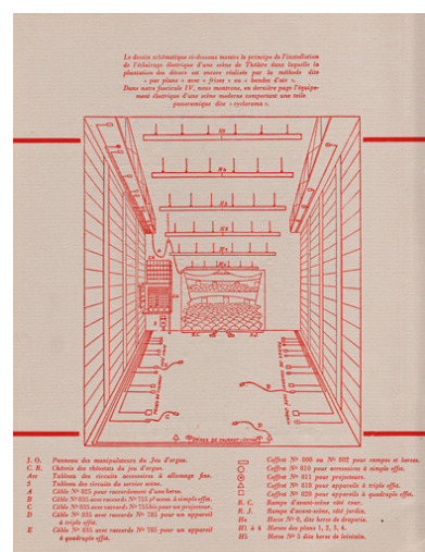
Cie générale de Travaux d'éclairage et de Force (Anciens Ets Cléménçon). Appareillages électriques pour théâtre [catalogue : principe d'installation
