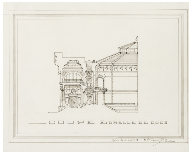
[Projet de cirque]. Coupe. 13 août 1903. Phot. Pierre-Marie Barbe- Richaud, Autr. Marcel Camuzat IVR26_20245800443NUC2A
