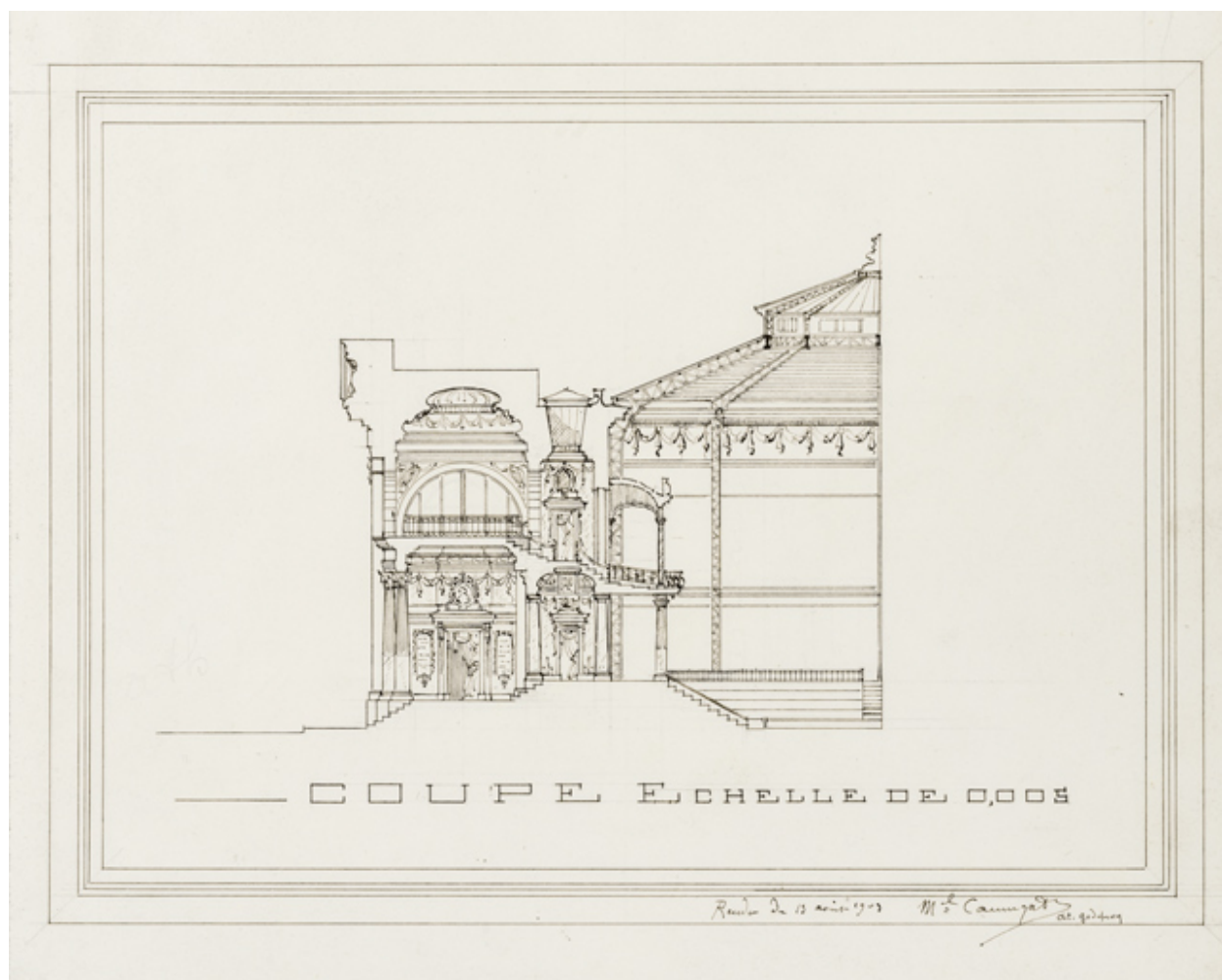
[Projet de cirque]. Coupe. 13 août 1903.
