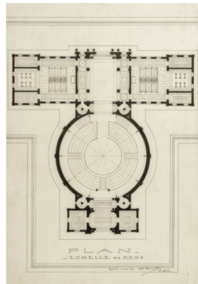
[Projet de cirque]. Plan. 13 août 1903.
