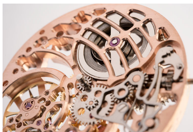
Mouvement rose, détail côté cadran : amortisseur de chocs (à gauche), tirette et pont de barillet (avec ressort moteur). Phot. Sonia Dourlot IVR43_20182501164NUC4A
