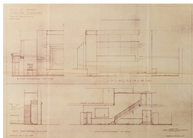
Théâtre municipal. Transformations. Coupes. 18 mai 1931. Phot. Pierre-Marie Barbe-Richaud, Autr. Marcel Dumontant, Autr. Marcel Bourgeon IVR26_20238900062NUC2A
