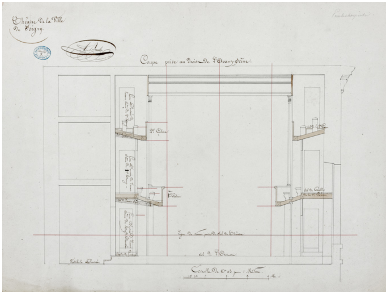
Construction de la salle de spectacle. Coupe prise au droit de l'avant-scène. Pour le charpentier. 1832.
