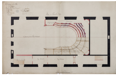
Construction de la salle de spectacle. Plan du 1er étage comprenant 1ères loges de face, 1ères loges de côté, 1ère galerie, balcon, 1ères loges d'avant-scène. 1832. Phot. Pierre-Marie Barbe-Richaud, Autr. Alexandre Bourla IVR26_20238900072NUC4A
