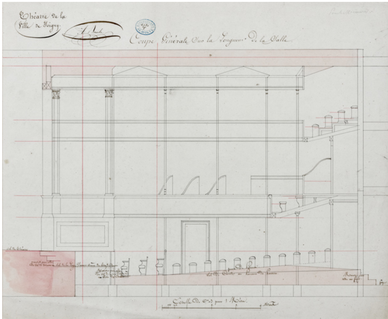
Construction de la salle de spectacle. Coupe générale sur la longueur de la salle. Pour le menuisier. 1832.
