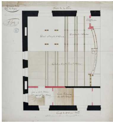
Construction de la salle de spectacle. Détails de la scène. Pour le menuisier machiniste. 1832. Phot. Pierre-Marie Barbe-Richaud, Autr. Alexandre Bourla IVR26_20238900081NUC2A
