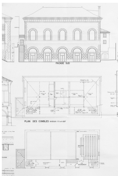
Réaménagement de l'ancien théâtre. Plans - coupes - façades. Etat des lieux [détail : façade sud et plans]. 6 décembre 1992. Phot. Pierre-Marie Barbe-Richaud, Autr. Didier Michelin IVR26_20238900050NUC4A
