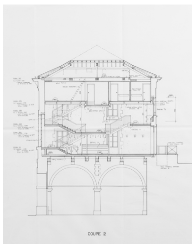
Réaménagement de l'ancien théâtre. Coupes 2-3. [Détail :] Coupe 2. Septembre 1994. Phot. Pierre-Marie Barbe-Richaud, Autr. Didier Michelon IVR26_20238900057NUC4A
