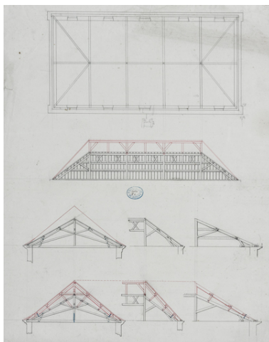
[Plan et coupes de la charpente]. S.d. [1859 ?]. Phot. Pierre-Marie Barbe-Richaud, Autr. A. Benoît IVR26_20238900095NUC2A
