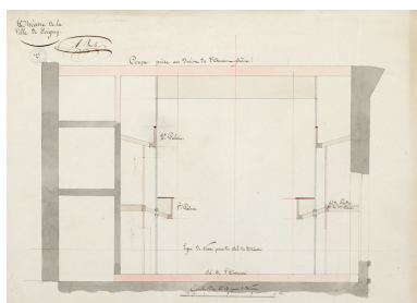
Construction de la salle de spectacle. Coupe prise au droit de l'avant-scène. Pour le menuisier. 1832. Phot. Pierre-Marie Barbe-Richaud, Autr. Alexandre Bourla IVR26_20238900094NUC4A
