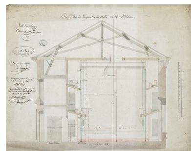
Construction de la salle de spectacle. Coupe sur la largeur de la salle côté du rideau. Pour la Ville de Joigny. 1832. Phot. Pierre-Marie Barbe-Richaud, Autr. Alexandre Bourla IVR26_20238900092NUC4A
