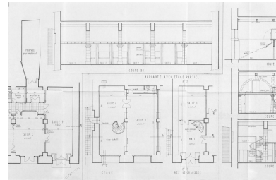
Projet d'aménagement de l'ancienne halle aux grains. [Détail :] Variante avec étage partiel [et] Coupe BB. Mai-juin 1980. Phot. Pierre-Marie Barbe-Richaud, Autr. Davy et Zanetta Architectes IVR26_20238900048NUC4A
