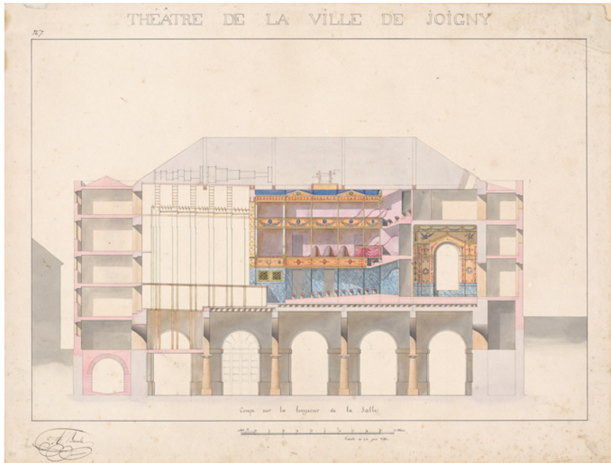
Coupe sur la longueur de la salle. N° 7. S.d. [1829-1830]. (MAP : G/82/89/2008-039062)
