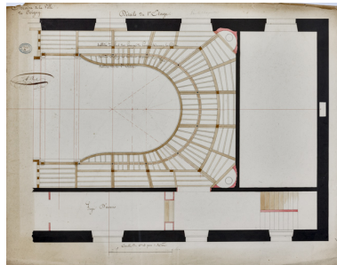
Construction de la salle de spectacle. Détail du 1er étage. Pour le charpentier. 1832. Phot. Pierre-Marie Barbe-Richaud, Autr. Alexandre Bourla IVR26_20238900078NUC2A
