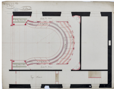
Construction de la salle de spectacle. [1er étage : loges et banquettes]. Pour le menuisier. 1832. Phot. Pierre-Marie Barbe-Richaud, Autr. Alexandre Bourla IVR26_20238900077NUC2A
