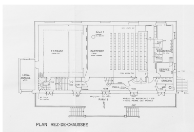
Réaménagement de l'ancien théâtre. Plans - coupes - façades. Etat des lieux. Plan rez-de-chaussée. 6 décembre 1992. Phot. Pierre-Marie Barbe-Richaud, Autr. Didier Michelin IVR26_20238900051NUC4A
