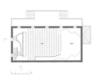
Plan de l'étage carré. D'après un plan non daté fourni par les Services techniques de la Ville. Dess. Aline Thomas, Autr. auteur inconnu IVR26_20238900767NUDA
