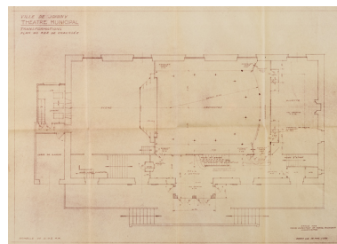
Théâtre municipal. Transformations. Plan du rez-de-chaussée. 18 mai 1931. Phot. Pierre-Marie Barbe-Richaud, Autr. Marcel Dumontant, Autr. Marcel Bourgeon IVR26_20238900064NUC2A
