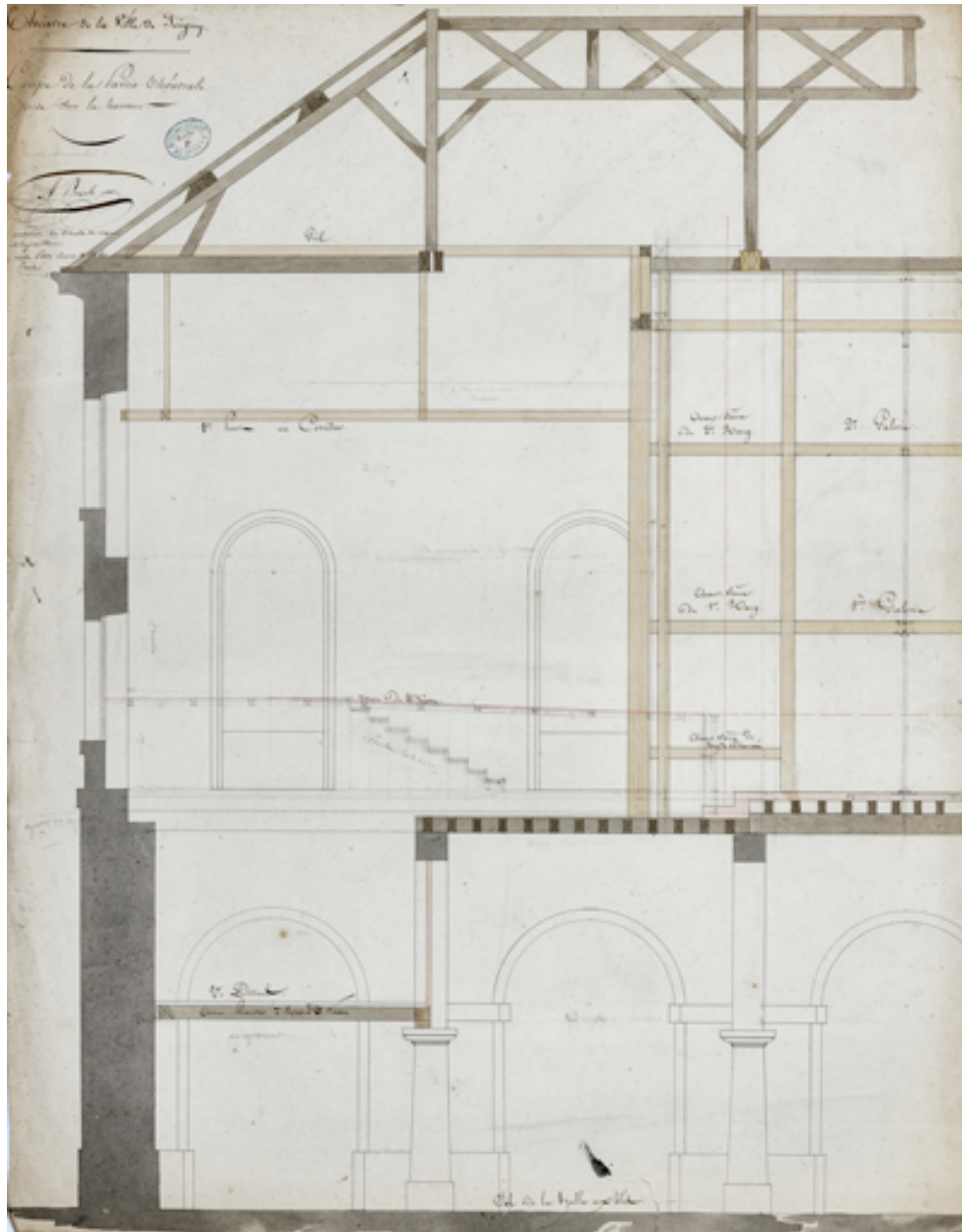
Construction de la salle de spectacle. Coupe de la partie théâtrale prise sur la hauteur. Pour le charpentier. 1832.
