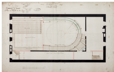
Construction de la salle de spectacle. Plan et détails du 2e étage. 1832. Phot. Pierre-Marie Barbe-Richaud, Autr. Alexandre Bourla IVR26_20238900074NUC4A
