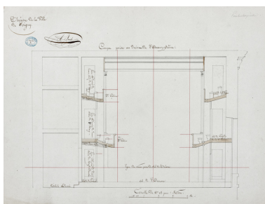
Construction de la salle de spectacle. Coupe prise au droit de l'avant-scène. Pour le charpentier. 1832. Phot. Pierre-Marie Barbe-Richaud, Autr. Alexandre Bourla IVR26_20238900093NUC4A
