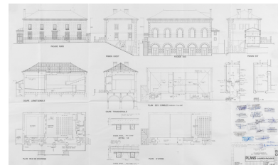
Réaménagement de l'ancien théâtre. Plans - coupes - façades. Etat des lieux. 6 décembre 1992. Phot. Pierre-Marie Barbe- Richaud, Autr. Didier Michelin IVR26_20238900049NUC4A
