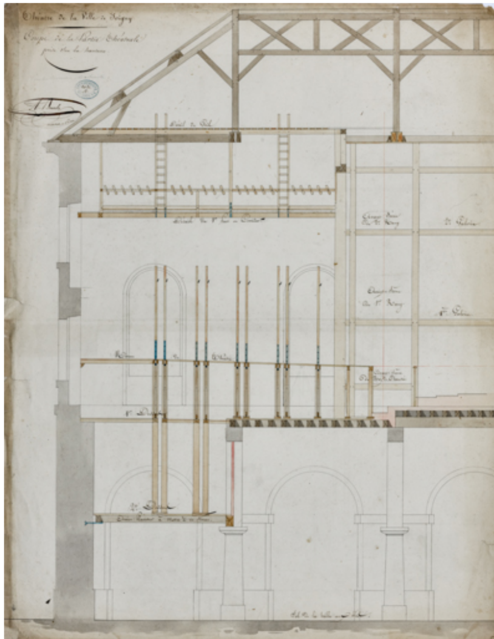
Construction de la salle de spectacle. Coupe de la partie théâtrale prise sur la hauteur [avec dessin des machines]. Pour le menuisier machiniste. 1832.
