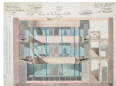
Construction de la salle de spectacle. Coupe sur la largeur de la salle. Pour la Ville de Joigny. 1832. Phot. Pierre-Marie Barbe-Richaud, Autr. Alexandre Bourla IVR26_20238900089NUC4A
