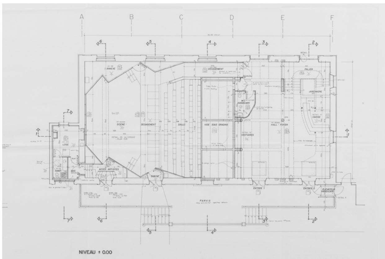
Réaménagement de l'ancien théâtre. Plan RdC 0.00. Septembre 1994.
