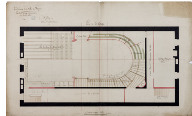
Construction de la salle de spectacle. Plan du 2e étage, amphithéâtre et 2e avant-scène. 1832. Phot. Pierre-Marie Barbe-Richaud, Autr. Alexandre Bourla IVR26_20238900073NUC4A
