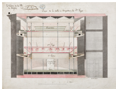
Construction de la salle de spectacle. Coupe de la salle en regardant les 1ères loges. 1832. Phot. Pierre-Marie Barbe-Richaud, Autr. Alexandre Bourla IVR26_20238900088NUC4A
