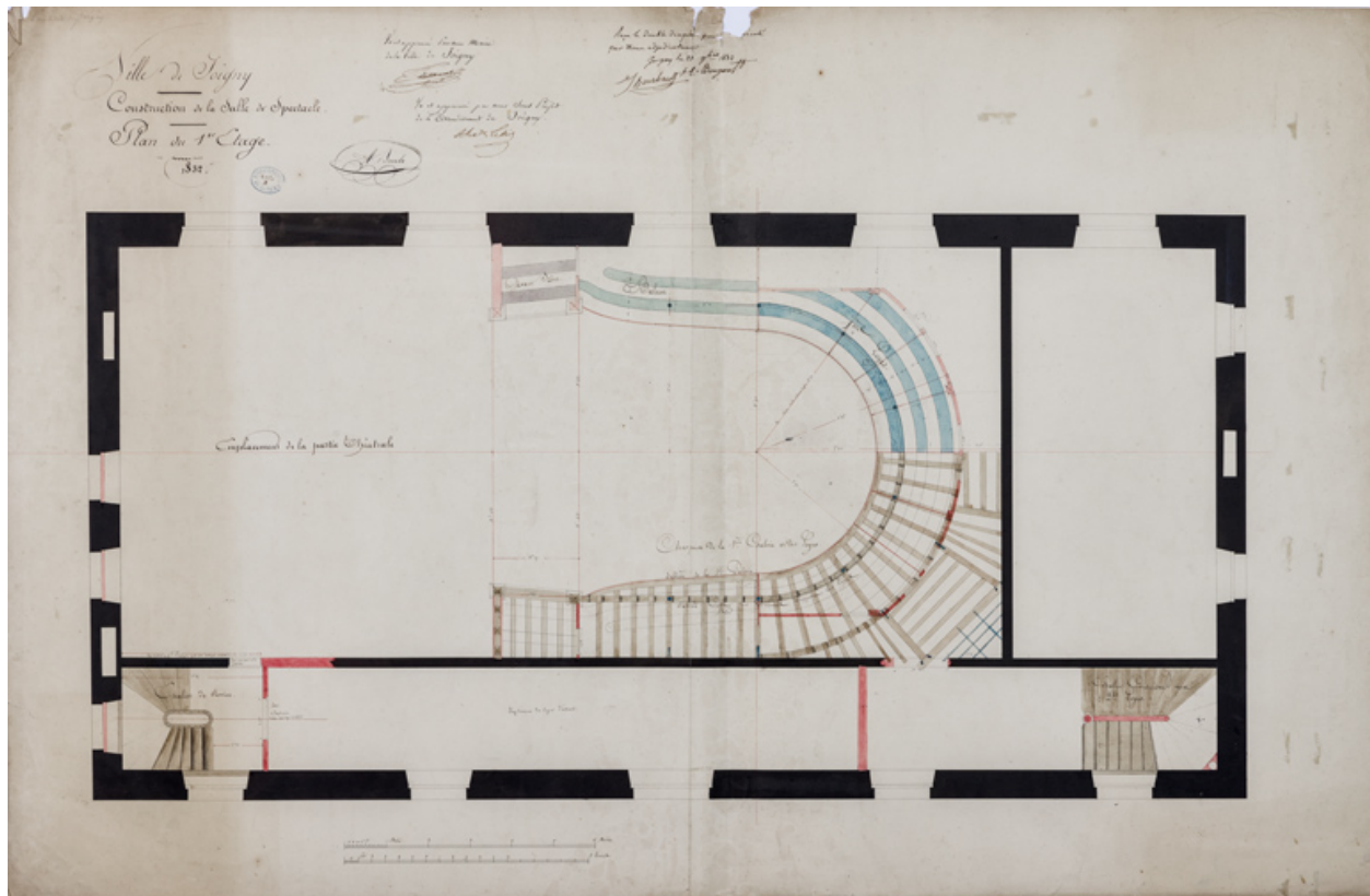
Construction de la salle de spectacle. Plan du 1er étage. 1832.
