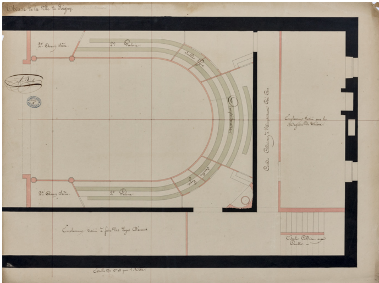
Construction de la salle de spectacle. [2e étage : loges et banquettes]. Pour le menuisier. 1832.
