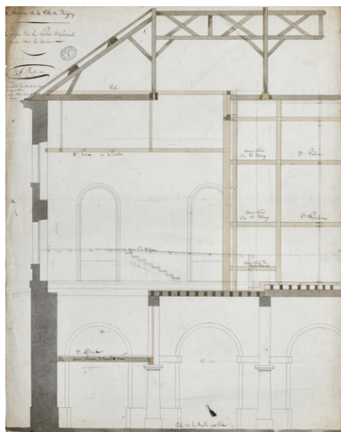
Construction de la salle de spectacle. Coupe de la partie théâtrale prise sur la hauteur. Pour le charpentier. 1832. Phot. Pierre-Marie Barbe-Richaud, Autr. Alexandre Bourla IVR26_20238900090NUC4A
