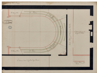
Construction de la salle de spectacle. [2e étage : loges et banquettes]. Pour le menuisier. 1832. Phot. Pierre-Marie Barbe-Richaud, Autr. Alexandre Bourla IVR26_20238900079NUC2A
