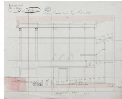
Construction de la salle de spectacle. Coupe générale sur la longueur de la salle. Pour le menuisier. 1832. Phot. Pierre-Marie Barbe-Richaud, Autr. Alexandre Bourla IVR26_20238900083NUC2A
