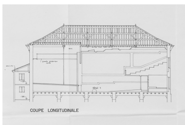
Réaménagement de l'ancien théâtre. Plans - coupes - façades. Etat des lieux. Coupe longitudinale. 6 décembre 1992. Phot. Pierre-Marie Barbe-Richaud, Autr. Didier Michelin IVR26_20238900055NUC4A
