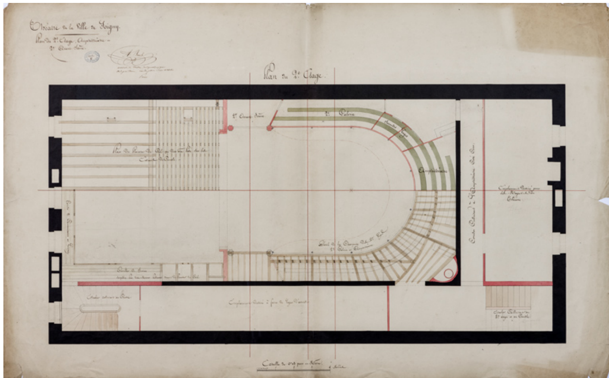
Construction de la salle de spectacle. Plan du 2e étage, amphithéâtre et 2e avant-scène. 1832.
