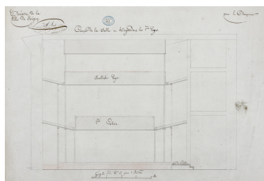
Construction de la salle de spectacle. Coupe de la salle en regardant les 1ères loges. Pour le charpentier. 1832. Phot. Pierre-Marie Barbe-Richaud, Autr. Alexandre Bourla IVR26_20238900086NUC4A
