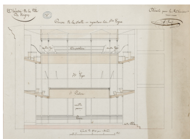
Construction de la salle de spectacle. Coupe de la salle en regardant les 1ères loges. Détails pour le menuisier. 1832. Phot. Pierre-Marie Barbe-Richaud, Autr. Alexandre Bourla IVR26_20238900087NUC4A
