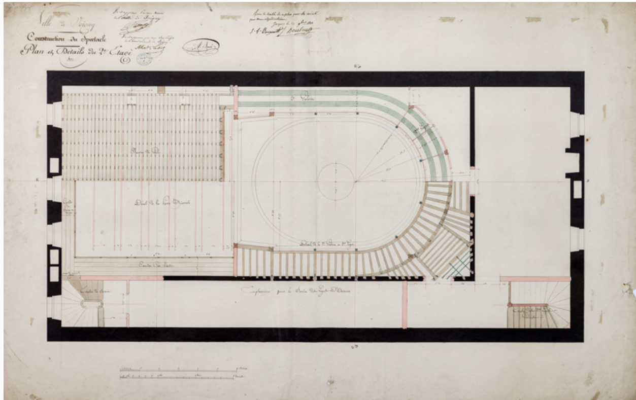
Construction de la salle de spectacle. Plan et détails du 2 e étage. 1832.
