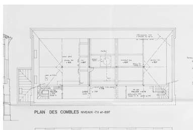
Réaménagement de l'ancien théâtre. Plans - coupes - façades. Etat des lieux. Plan des combles. 6 décembre 1992. Phot. Pierre-Marie Barbe-Richaud, Autr. Didier Michelin IVR26_20238900053NUC4A
