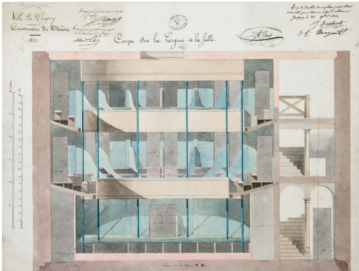
Construction de la salle de spectacle. Coupe sur la largeur de la salle. Pour la Ville de Joigny. 1832.
