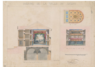
Coupe sur la largeur au droit de l'avant-scène, Coupe sur la largeur au droit des loges [et] Détail du plafond. N° 8. S.d. [1829-1830]. (MAP : G/82/89/2008-039064) Autr. Alexandre Bourla, Phot. Médiathèque du Patrimoine et de la Photographie IVR26_20238900105NUC4A
