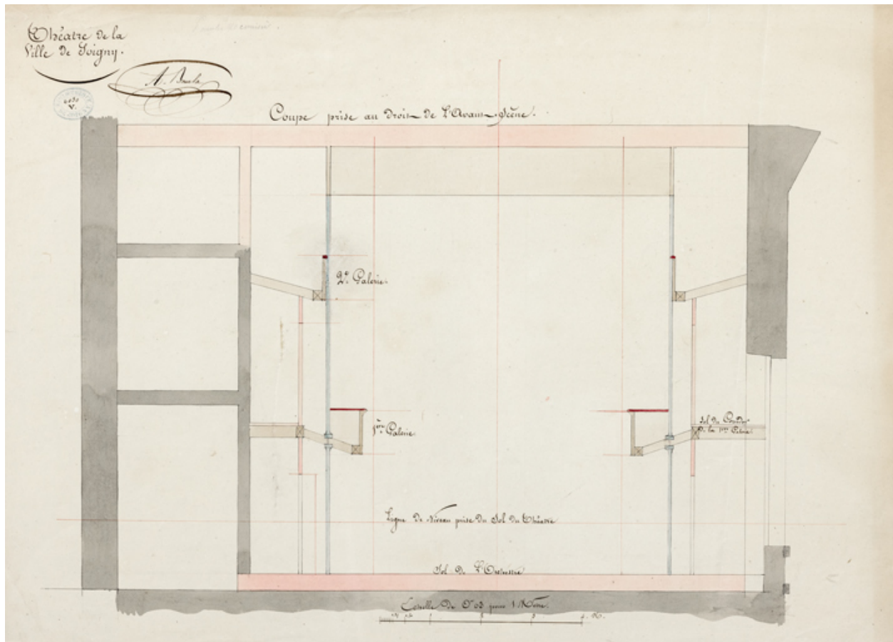
Construction de la salle de spectacle. Coupe prise au droit de l'avant-scène. Pour le menuisier. 1832.
