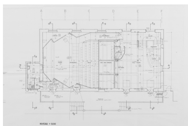
Réaménagement de l'ancien théâtre. Plan RdC 0.00. Septembre 1994. Phot. Pierre-Marie Barbe-Richaud, Autr. Didier Michelin IVR26_20238900059NUC4A
