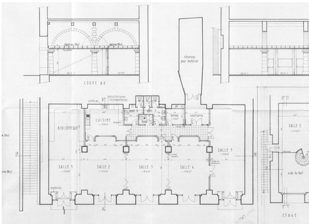
Projet d'aménagement de l'ancienne halle aux grains. [Détail : plan et] Coupe AA. Mai-juin 1980.
