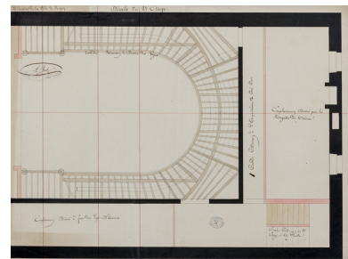
Construction de la salle de spectacle. Détail du 2e étage. Pour le charpentier. 1832. Phot. Pierre-Marie Barbe-Richaud, Autr. Alexandre Bourla IVR26_20238900080NUC2A
