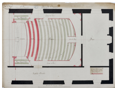
Construction de la salle de spectacle. Rez de chaussée. Pour le menuisier. 1832. Phot. Pierre-Marie Barbe- Richaud, Autr. Alexandre Bourla IVR26_20238900075NUC4A
