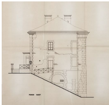
Réaménagement de l'ancien théâtre. Etat actuel. Pignons [pignon ouest]. 17 mai 1988. Phot. Pierre-Marie Barbe- Richaud, Autr. Didier Michelin IVR26_20238900066NUC2A
