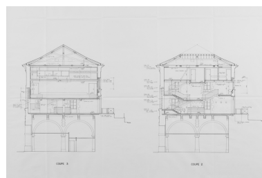
Réaménagement de l'ancien théâtre. Coupes 2-3. Septembre 1994. Phot. Pierre-Marie Barbe-Richaud, Autr. Didier Michelin IVR26_20238900056NUC4A
