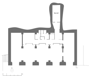
Plan de l'étage de soubassement. D'après un plan non daté fourni par les Services techniques de la Ville. Dess. Aline Thomas, Autr. auteur inconnu IVR26_20238900766NUDA
