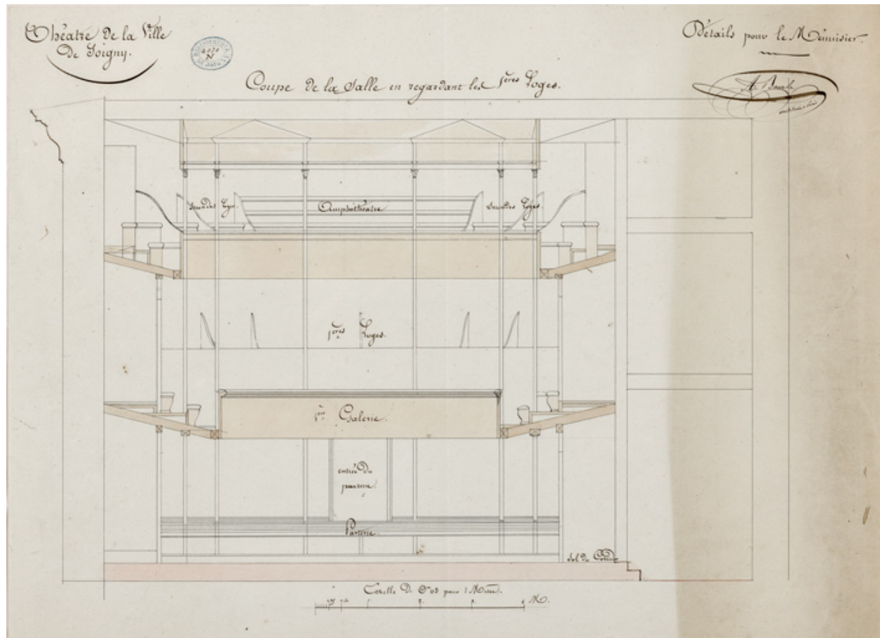
Construction de la salle de spectacle. Coupe de la salle en regardant les 1ères loges. Détails pour le menuisier. 1832.
