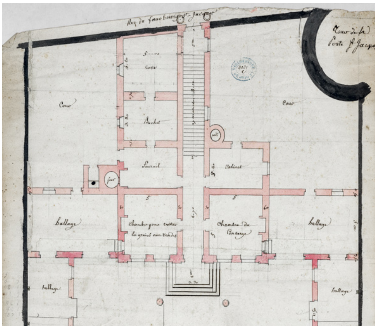
Plan des bâtimens, hallages, places & du marché à blé de Joigny projeté sur le terrain de la Petite Bute [... Détail du bâtiment]. 18 avril 1817.
