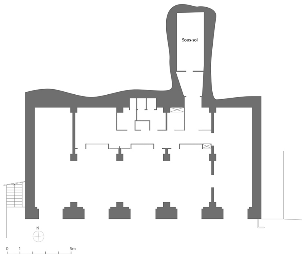
Plan de l'étage de soubassement. D'après un plan non daté fourni par les Services techniques de la Ville.
