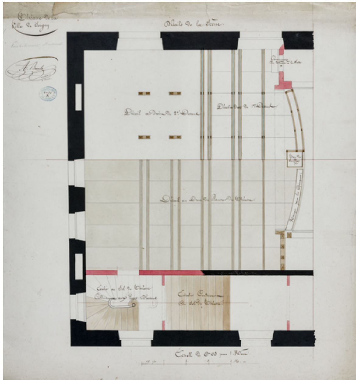
Construction de la salle de spectacle. Détails de la scène. Pour le menuisier machiniste. 1832.
