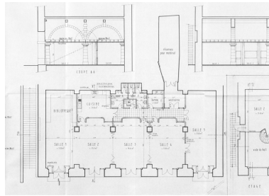
Projet d'aménagement de l'ancienne halle aux grains. [Détail : plan et] Coupe AA. Mai-juin 1980. Phot. Pierre-Marie Barbe-Richaud, Autr. Davy et Zanetta Architectes IVR26_20238900047NUC4A
