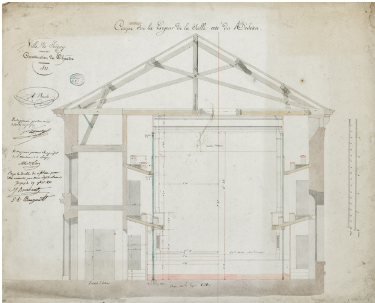
Construction de la salle de spectacle. Coupe sur la largeur de la salle côté du rideau. Pour la Ville de Joigny. 1832.
