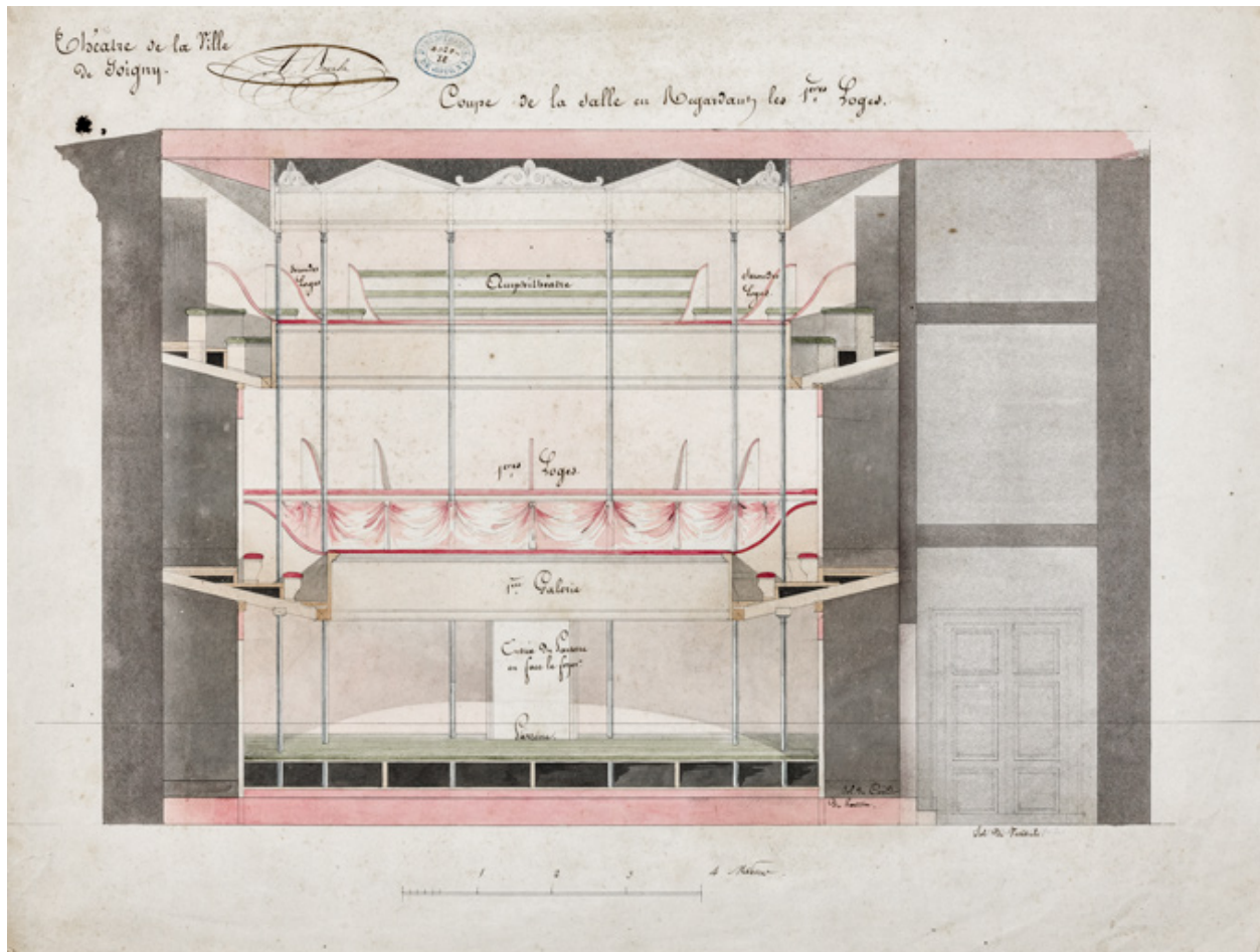
Construction de la salle de spectacle. Coupe de la salle en regardant les 1ères loges. 1832.
