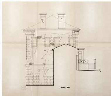
Réaménagement de l'ancien théâtre. Etat actuel. Pignons [pignon est]. 17 mai 1988. Phot. Pierre-Marie Barbe- Richaud, Autr. Didier Michelin IVR26_20238900067NUC2A
