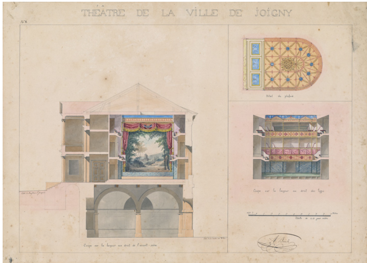
Coupe sur la largeur au droit de l'avant-scène, Coupe sur la largeur au droit des loges [et] Détail du plafond. N° 8. S.d. [1829-1830]. (MAP : G/82/89/2008-039064)
