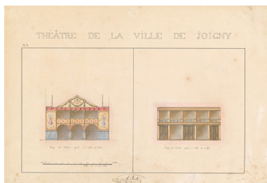
Coupe du théâtre ajusté en salle de bal [et] Coupe du théâtre ajusté en salle de vente. N° 9. S.d. [1829-1830]. (MAP : G/82/89/2008-039061) Autr. Alexandre Bourla, Phot. Médiathèque du Patrimoine et de la Photographie IVR26_20238900102NUC4A
