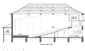
Coupe longitudinale. D'après une coupe non datée fournie par les Services techniques de la Ville. Dess. Aline Thomas, Autr. auteur inconnu IVR26_20238900768NUDA
