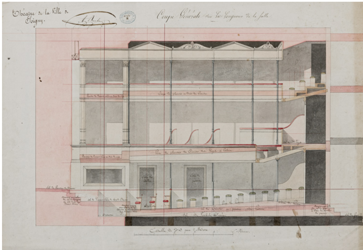
Construction de la salle de spectacle. Coupe générale sur la longueur de la salle. 1832.
