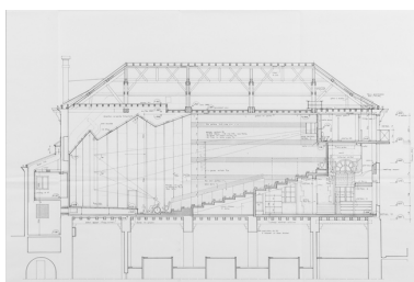
Réaménagement de l'ancien théâtre. Coupe 1. Septembre 1994. Phot. Pierre-Marie Barbe-Richaud, Autr. Didier Michelin IVR26_20238900058NUC4A
