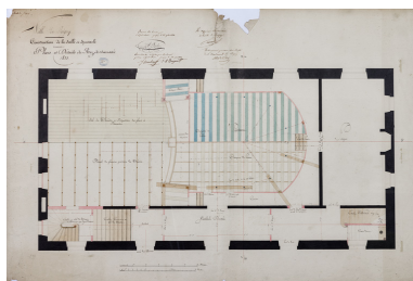
Construction de la salle de spectacle. Plan et détails du rez-de-chaussée. 1832. Phot. Pierre-Marie Barbe- Richaud, Autr. Alexandre Bourla IVR26_20238900070NUC4A
