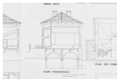
Réaménagement de l'ancien théâtre. Plans - coupes - façades. Etat des lieux. Coupe transversale. 6 décembre 1992. Phot. Pierre-Marie Barbe-Richaud, Autr. Didier Michelin IVR26_20238900054NUC4A
