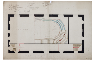
Construction de la salle de spectacle. Plan du 1er étage. 1832. Phot. Pierre-Marie Barbe-Richaud, Autr. Alexandre Bourla IVR26_20238900071NUC4A
