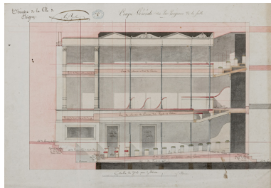
Construction de la salle de spectacle. Coupe générale sur la longueur de la salle. 1832. Phot. Pierre-Marie Barbe-Richaud, Autr. Alexandre Bourla IVR26_20238900084NUC4A
