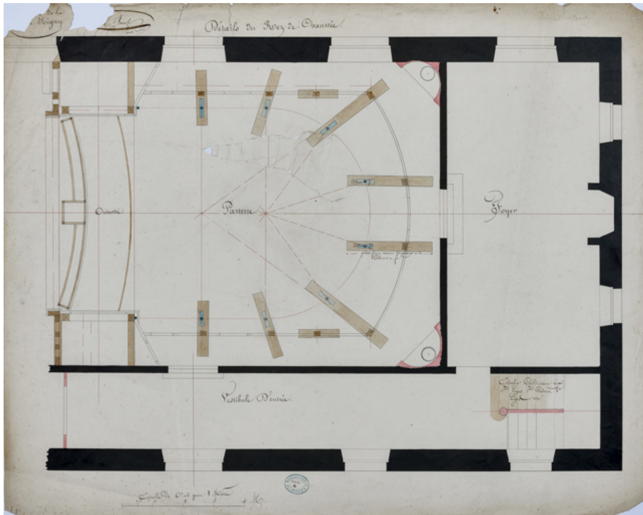
Construction de la salle de spectacle. Détails du rez de chaussée. Pour le charpentier. 1832.
