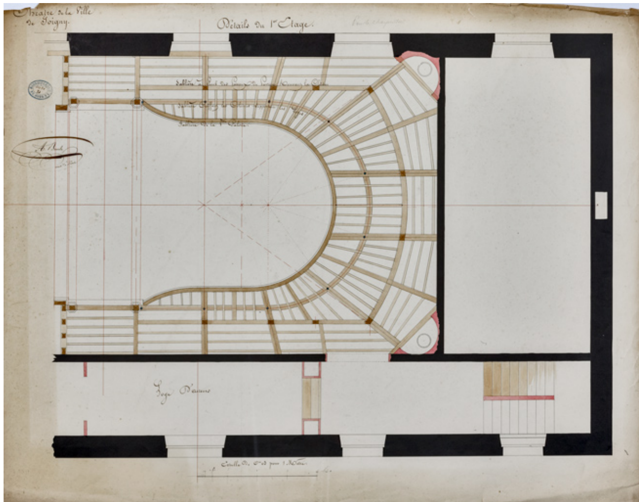
Construction de la salle de spectacle. Détail du 1er étage. Pour le charpentier. 1832.
