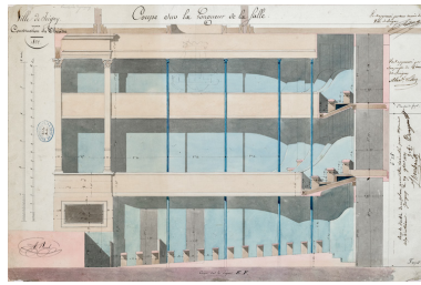
Construction de la salle de spectacle. Coupe sur la longueur de la salle. Pour la Ville de Joigny. 1832. Phot. Pierre-Marie Barbe-Richaud, Autr. Alexandre Bourla IVR26_20238900085NUC4A
