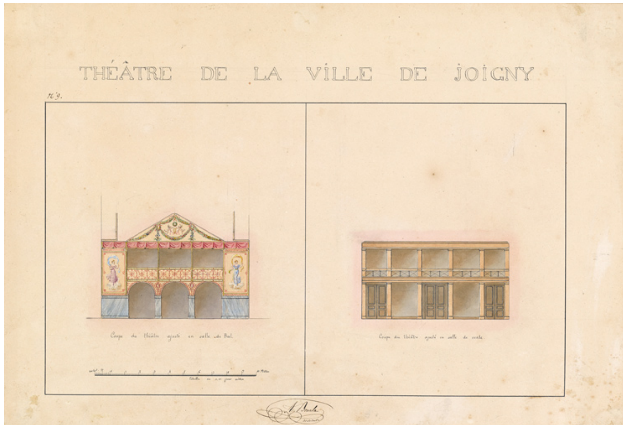
Coupe du théâtre ajusté en salle de bal [et] Coupe du théâtre ajusté en salle de vente. N° 9. S.d. [1829-1830]. (MAP : G/82/89/2008-039061)
