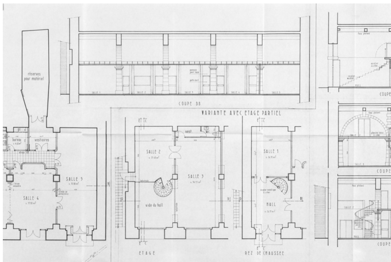
Projet d'aménagement de l'ancienne halle aux grains. [Détail :] Variante avec étage partiel [et] Coupe BB. Mai-juin 1980.
