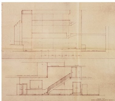
Théâtre municipal. Transformations. Coupes [détail]. 18 mai 1931.
