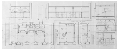
Projet d'aménagement de l'ancienne halle aux grains. Mai-juin 1980. Phot. Pierre-Marie Barbe-Richaud, Autr. Davy et Zanetta Architectes IVR26_20238900046NUC2A
