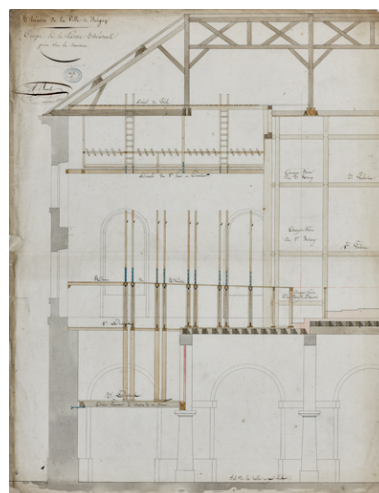
Construction de la salle de spectacle. Coupe de la partie théâtrale prise sur la hauteur [avec dessin des machines]. Pour le menuisier machiniste. 1832. Phot. Pierre-Marie Barbe-Richaud, Autr. Alexandre Bourla IVR26_20238900091NUC4A
