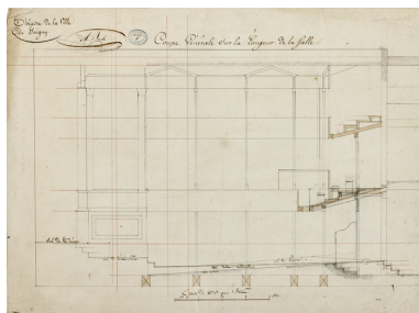
Construction de la salle de spectacle. Coupe générale sur la longueur [sic] de la salle. Pour le charpentier. 1832. Phot. Pierre-Marie Barbe-Richaud, Autr. Alexandre Bourla IVR26_20238900082NUC2A
