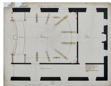
Construction de la salle de spectacle. Détails du rez de chaussée. Pour le charpentier. 1832. Phot. Pierre-Marie Barbe- Richaud, Autr. Alexandre Bourla IVR26_20238900076NUC2A
