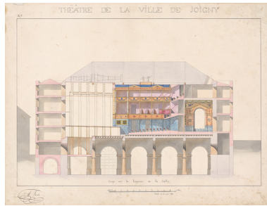
Coupe sur la longueur de la salle. N° 7. S.d. [1829-1830]. (MAP : G/82/89/2008-039062) Autr. Alexandre Bourla, Phot. Médiathèque du Patrimoine et de la Photographie IVR26_20238900103NUC4A
