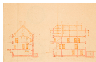
Commune de Fessevillers. Projet de construction d'une fruitière [détail : coupes], 1932. Phot. Jérôme Mongreville, Autr. Camille André IVR43_20152500561NUC4A
