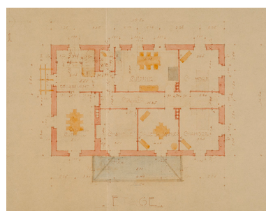
Commune de Fessevillers. Projet de construction d'une fruitière. Plans. Etage, 1932. Phot. Sonia Dourlot, Autr. Camille André IVR43_20152500471NUC4A
