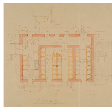
Commune de Fessevillers. Projet de construction d'une fruitière. Plans. Sous-sol, 1932. Phot. Sonia Dourlot, Autr. Camille André IVR43_20152500469NUC4A
