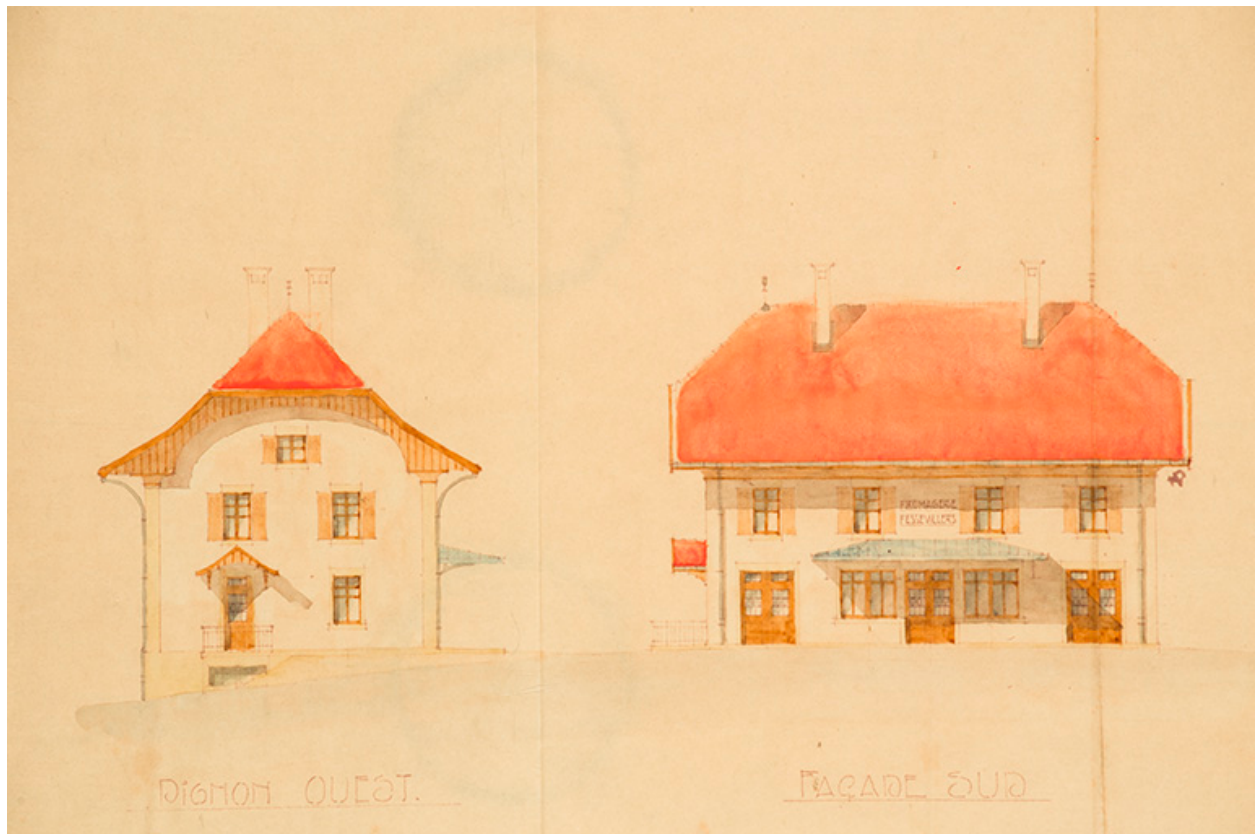
Commune de Fessevillers. Projet de construction d'une fruitière [détail : façades ouest et sud], 1932.
