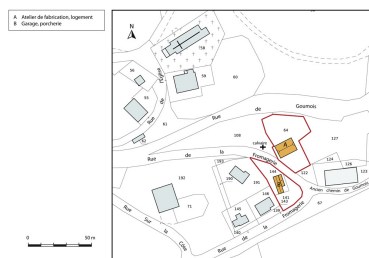
Plan-masse et de situation. Extrait du plan cadastral, 2013, section AB. Dess. Mathias Papigny IVR43_20142501540NUDA
