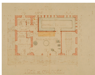
Commune de Fessevillers. Projet de construction d'une fruitière. Plans. Rez-de-chaussée, 1932. Phot. Sonia Dourlot, Autr. Camille André IVR43_20152500470NUC4A
