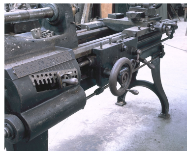
Détail de la boîte de vitesses et de la commande manuelle. Phot. Yves Sancey IVR43_20022500895XA
