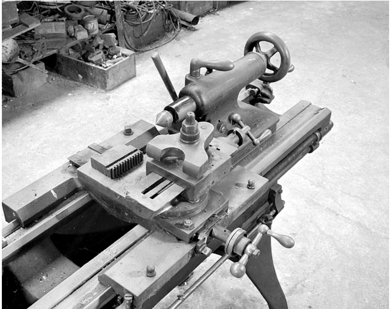
Détail du trainard et de la poupée mobile.
