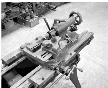
Détail du traînard et de la poupée mobile. Phot. Yves Sancey IVR43_20022500873X
