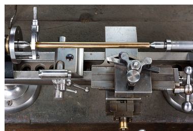
Grand tour : partie travaillante (barre entre pointe et contre- pointe à l'arrière-plan, support de lime à gauche et chariot porte-burin à droite). Phot. Sonia Dourlot IVR43_20172500132NUC4A
