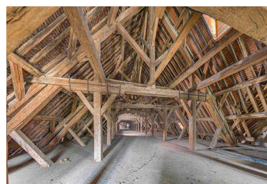
Charpente des grandes halles. Phot. Thierry Kuntz IVR26_20232100396NUC4A
