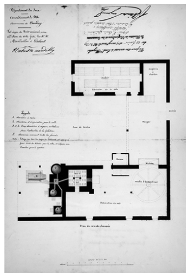
Fabrique de noir animal avec addition de colle forte par MM Mandrillon et Dubant. Plan du rez-de-chaussée.
