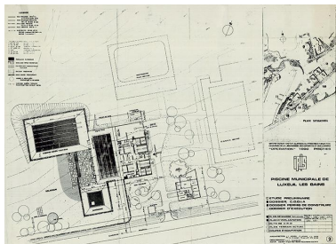
Plan-masse et de situation. IVR43_20267000072NUC4A
