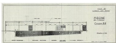
Coupe longitudinale de la piscine sur le bassin. IVR43_20267000067NUC4A
