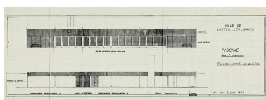
Élévations des faces nord- est (entrée) et nord-ouest. IVR43_20267000069NUC4A
