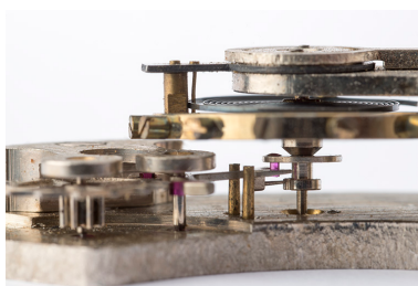
L'échappement : plateau du balancier muni de l'ellipse (cheville en rubis) engagée dans la fourchette de l'ancre. Le mouvement de cette dernière, dont le dard est visible au-dessous, est limité par les deux goupilles en laiton.
