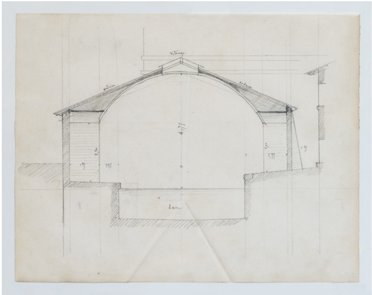
Piscine, projet, coupe transversale (vers 1866).
