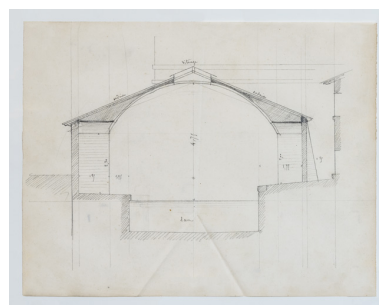
Piscine, projet, coupe transversale (vers 1866). Repro. Pierre-Marie Barbe- Richaud, Autr. Victor Petit IVR26_20195800338NUC2A
