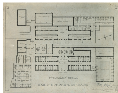
Projet de transformation et d'agrandissement (1899) de Gavillon, plan. Repro. Pierre-Marie Barbe- Richaud, Autr. Gavillon IVR26_20195800357NUC2A
