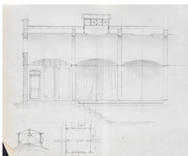
Piscine, projet, coupe longitudinale partielle (vers 1866). Repro. Pierre-Marie Barbe- Richaud, Autr. Victor Petit IVR26_20195800327NUC2A
