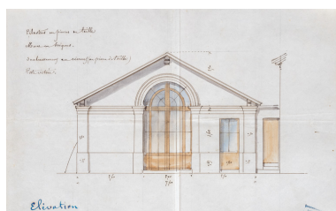
Piscine, projet, façade nord (vers 1866). Repro. Pierre-Marie Barbe- Richaud, Autr. Victor Petit IVR26_20195800328NUC2A
