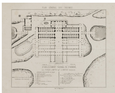
Plan de l'établissement thermal projeté avec les parties effectivement construites en 1854-1857. Phot. Pierre-Marie Barbe- Richaud, Autr. Jules François, Autr. Meyer, Autr. Andoche Parthiot IVR26_20195800343NUC2A
