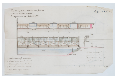
Piscine, projet, coupe longitudinale (vers 1866). Repro. Pierre-Marie Barbe- Richaud, Autr. Victor Petit IVR26_20195800336NUC4A
