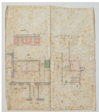
Projet de construction d'un bâtiment pour les bains de pieds (1882). Repro. Pierre-Marie Barbe- Richaud, Autr. auteur inconnu IVR26_20195800348NUC2A
