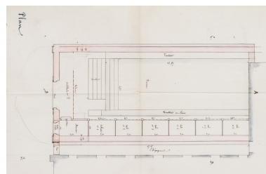
Piscine, projet, plan (vers 1866). Repro. Pierre-Marie Barbe- Richaud, Autr. Victor Petit IVR26_20195800334NUC2A
