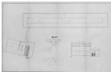
Plan dressé à l'appui d'une demande en autorisation d'établir divers appareils à vapeur dans le tissage de M. Winckler à Rougemont [plan et coupe longitudinale de la salle de la machine à vapeur]. Phot. Jérôme Mongreville IVR43_20019000020V
