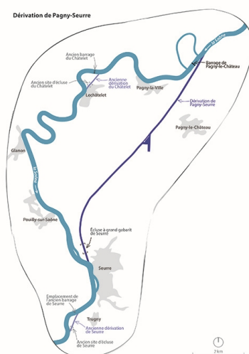
Plan schématique de la dérivation de Pagny-Seurre, échelle 1 / 5 000e. Dess. Aline Thomas IVR26_20222100183NUDA
