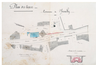
Plan de situation de la conduite d'assainissement à construire Phot. Jérôme Mongreville IVR43_20167001559NUC4A
