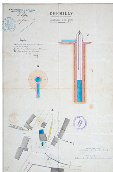
Plan de situation et plan en coupe du puits à reconstruire, 1865 Phot. Jérôme Mongreville IVR43_20167001551NUC4A
