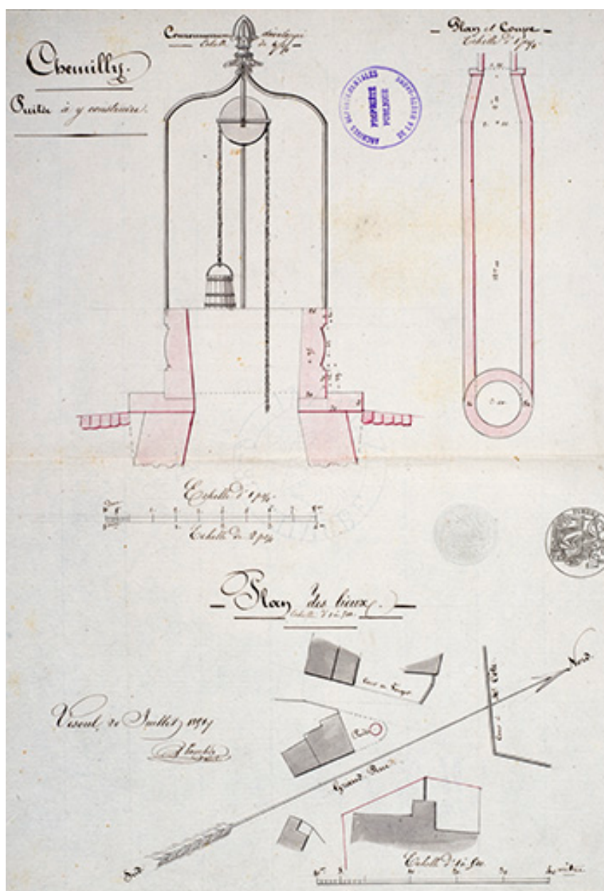
Plan du puits à reconstruire, 1851
