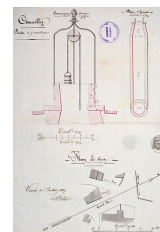
Plan du puits à reconstruire, 1851
