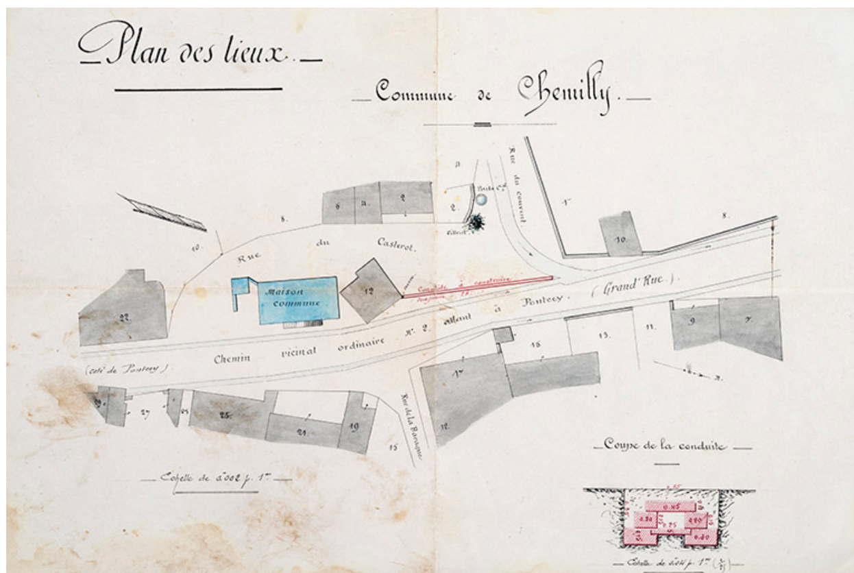
Plan de situation de la conduite d'assainissement à construire
