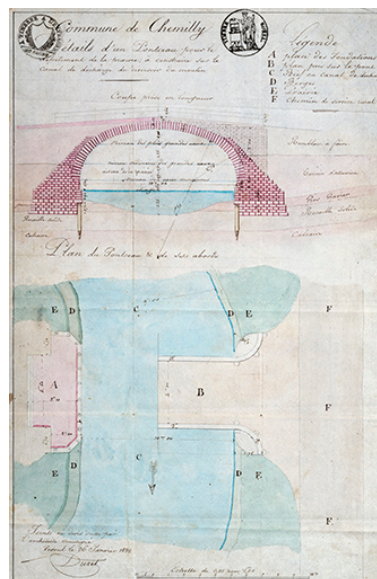
Plans du ponceau à construire, pour le défrichement de la prairie, sur le canal de décharge du déversoir du moulin, 1832 Phot. Jérôme Mongreville IVR43_20167001558NUC4A
