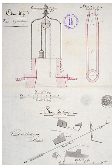
Plan du puits à reconstruire, 1851 Phot. Jérôme Mongreville IVR43_20167001552NUC4A
