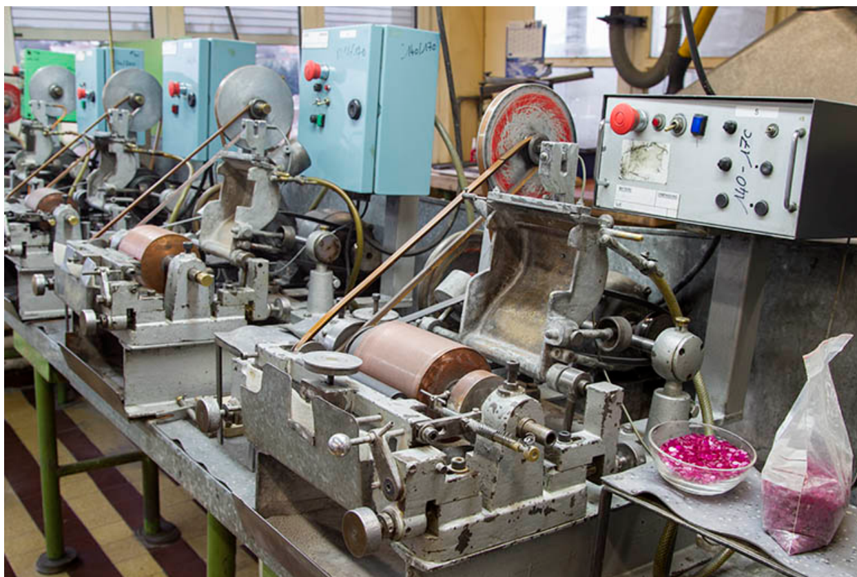
Atelier de taille du rubis : machines à usiner par abrasion (machines suisses Bocadero).
