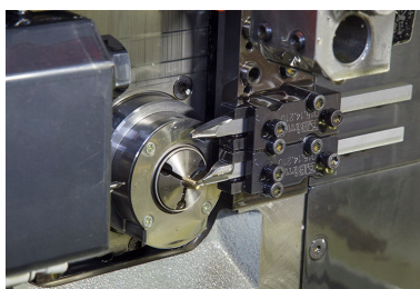
Machine à décolleter récente : pièce et outils. Phot. Sonia Dourlot IVR43_20142501940NUC2A
