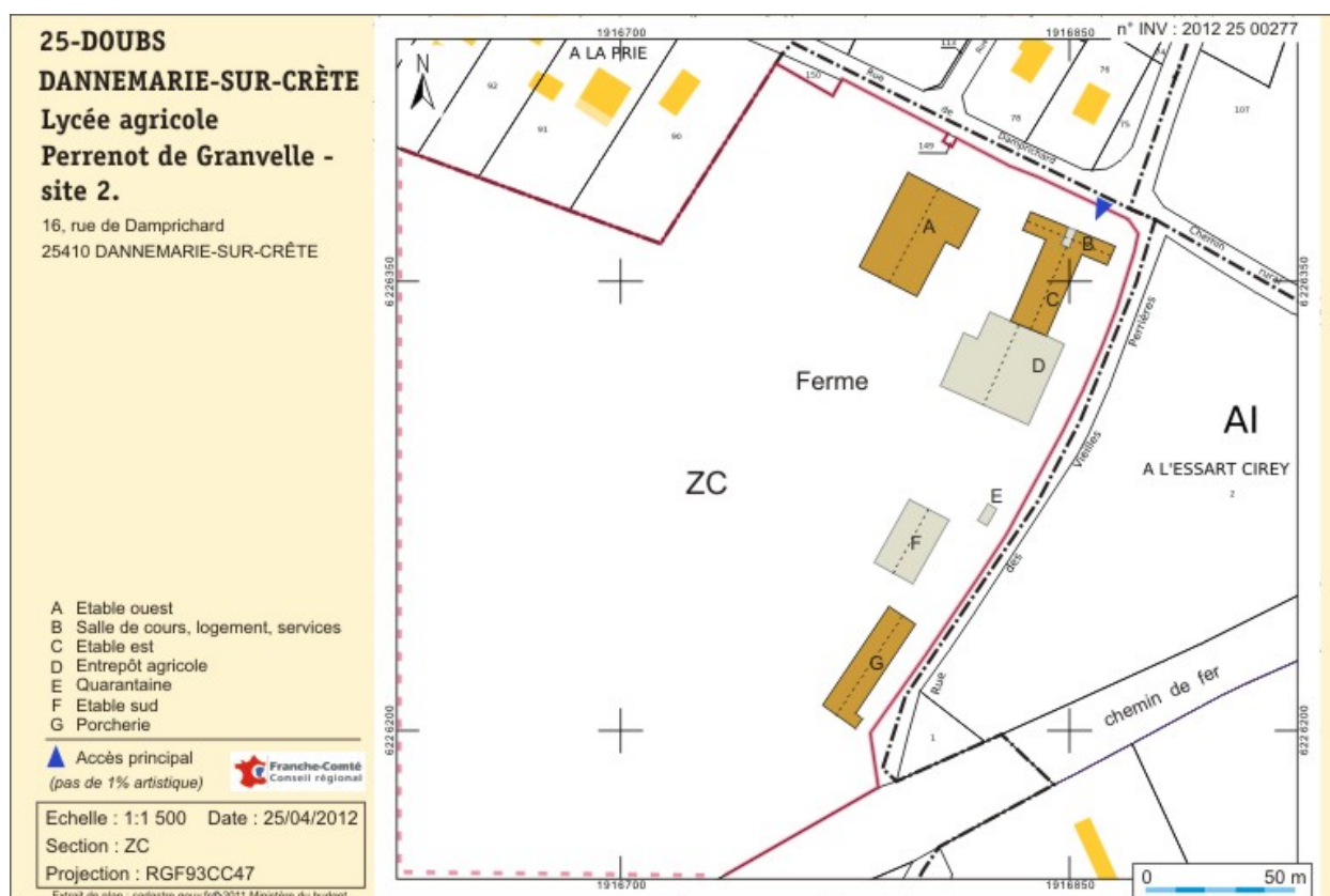
site 2 : plan-masse de la ferme d'application. Extrait du plan cadastral numérisé, 2011, section ZC, échelle 1:1500.
